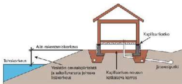
Kuva 11. Alin rakentamiskorkeus sokkeliperustukselle ja tuulettuvalle alapohjalle. Maanpinta ja etäisyys vesirajasta ovat määräävämpiä kuin kapillaarikatkon sijainti rakenteissa.
