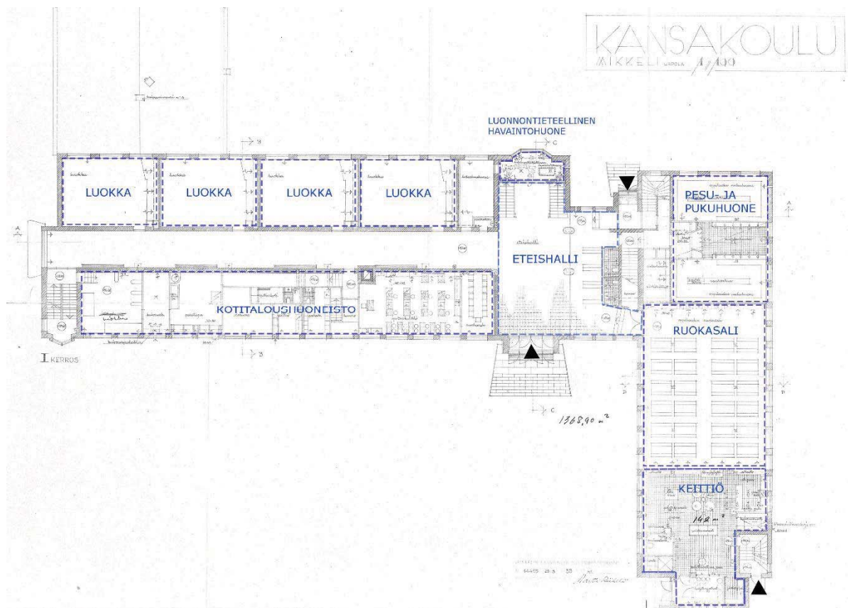
Ensimmäisen kerroksen pohjapiirustus. (Pohjapiirros Mikkelin rakennusvalvonta)
