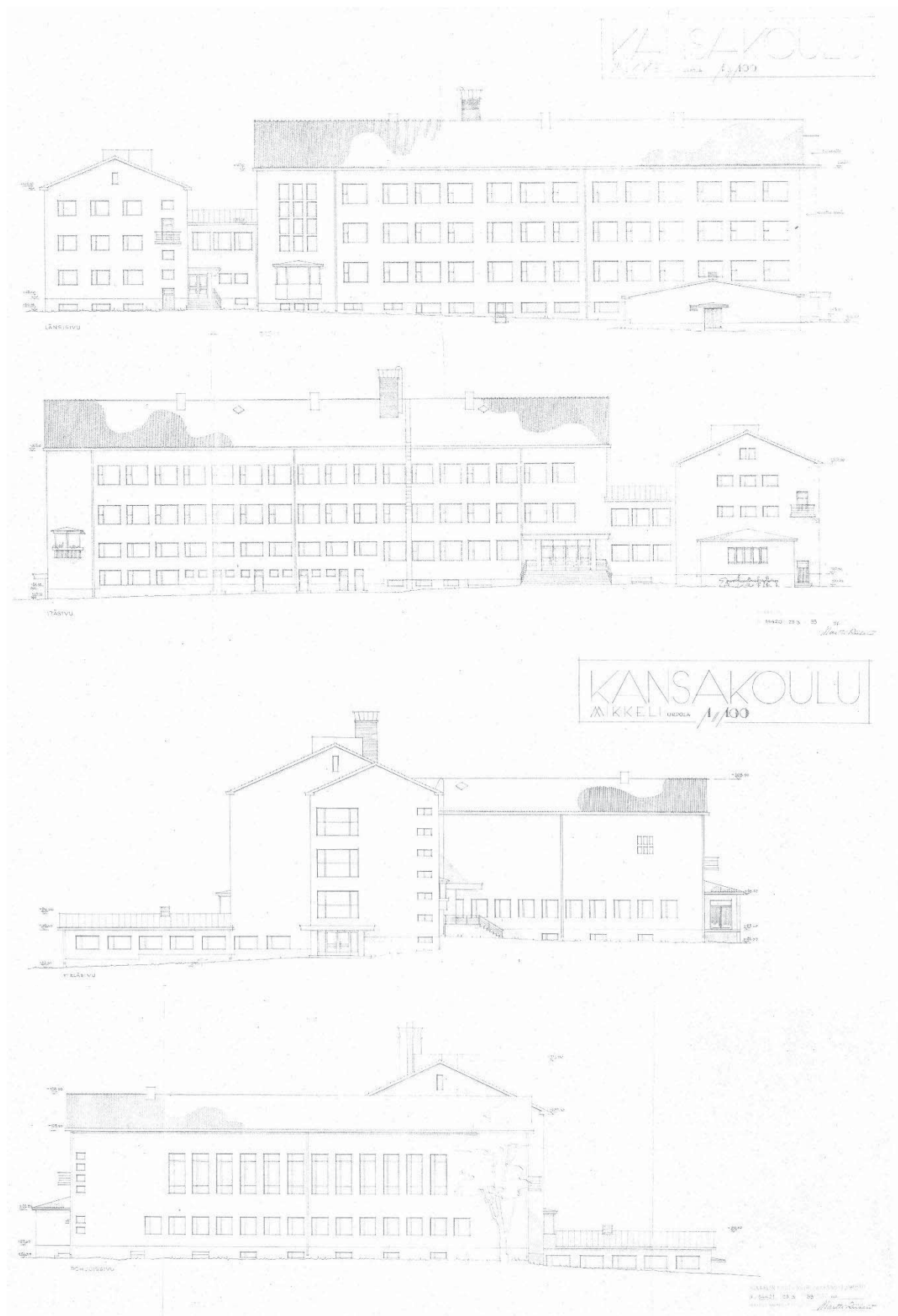
Urpolan kansakoulun julkisivupiirustukset vuodelta 1953. (Mikkelin rakennusvalvonta)
