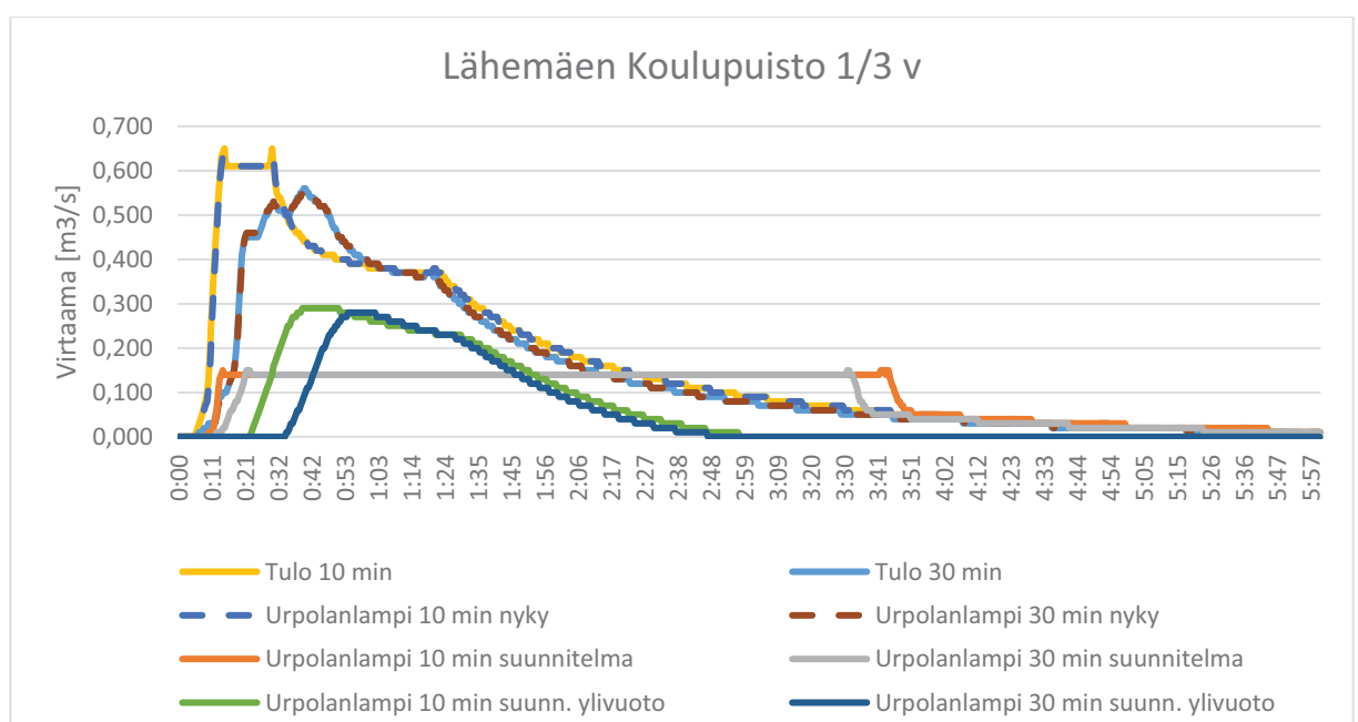
Kuva 1. Hulevesiverkoston virtausmallinnuksen tulokset suunnitellun kosteikon tulo- ja purkuvirtaamista
