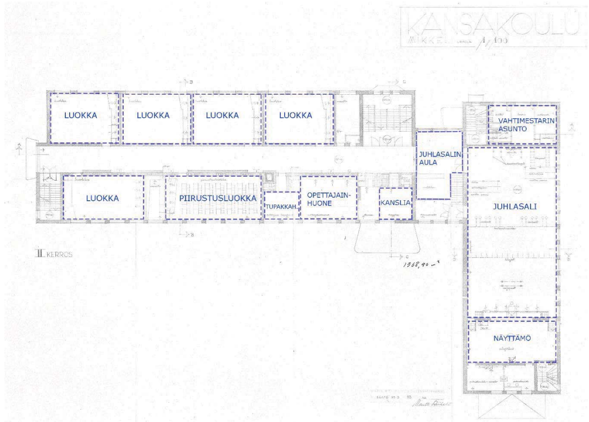
Toisen kerroksen pohjapiirustus. (Pohjapiirros Mikkelin rakennusvalvonta)
