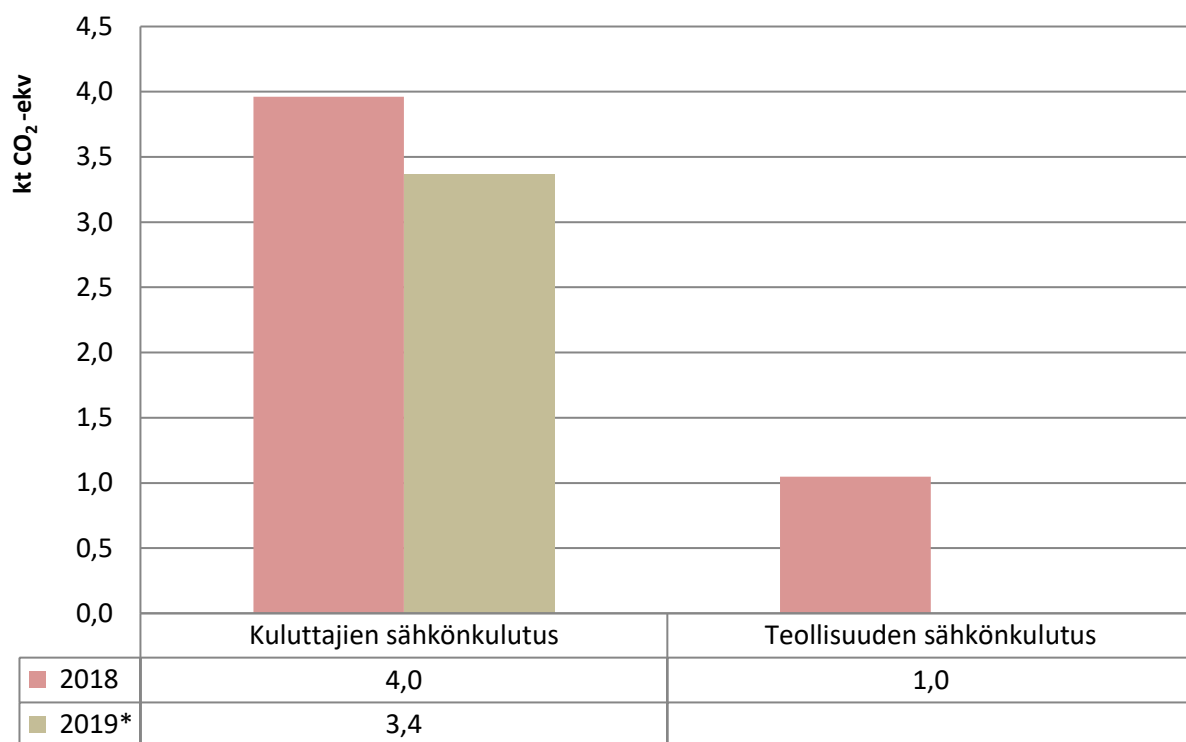
Kuva 3. Kuluttajien ja teollisuuden sähkönkulutuksen päästöjen kehitys Juvalla vuosina 2018–2019. Vuoden 2019 tieto on ennakkotieto. Sitä ei ole esitetty teollisuuden sähkönkulutukselle.
