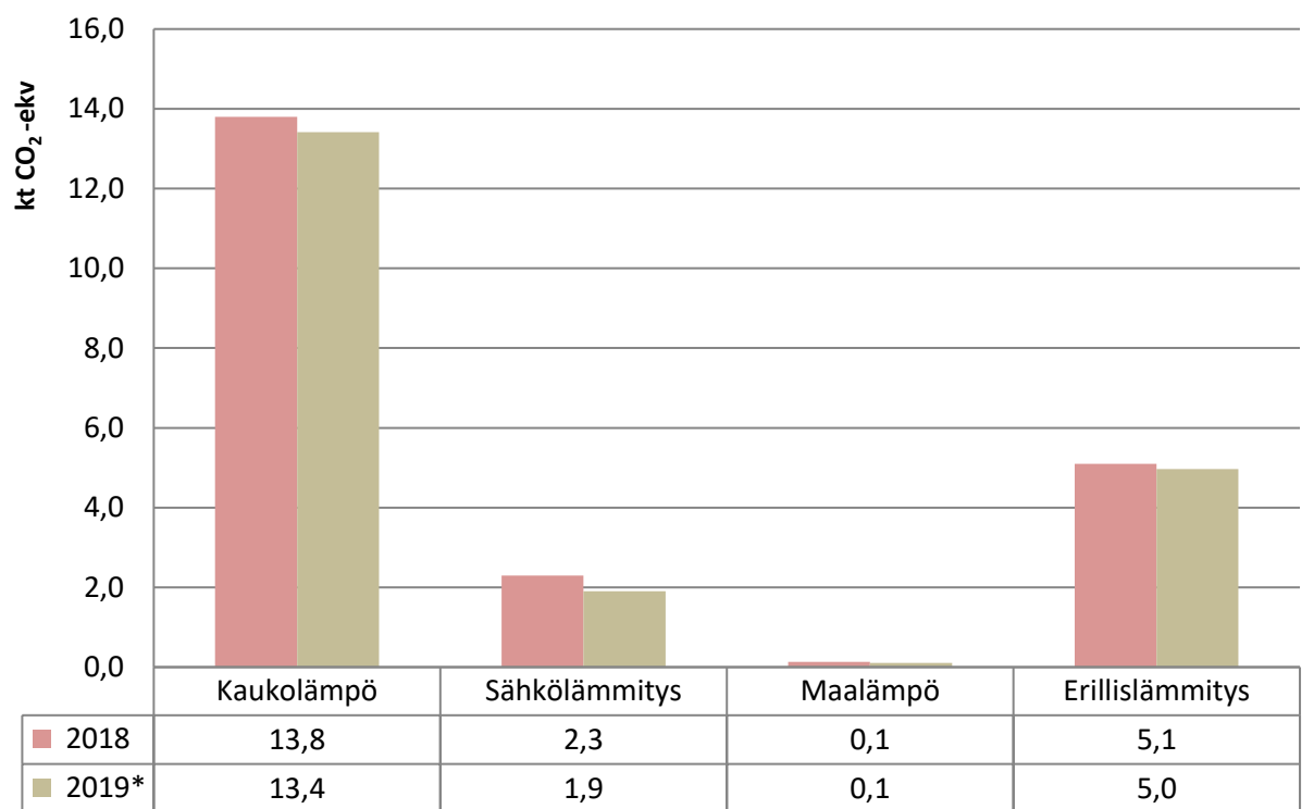
Kuva 6. Rakennusten lämmityksen päästöjen kehitys Juvalla vuosina 2018–2019. Vuoden 2019 tieto on ennakkotieto.
