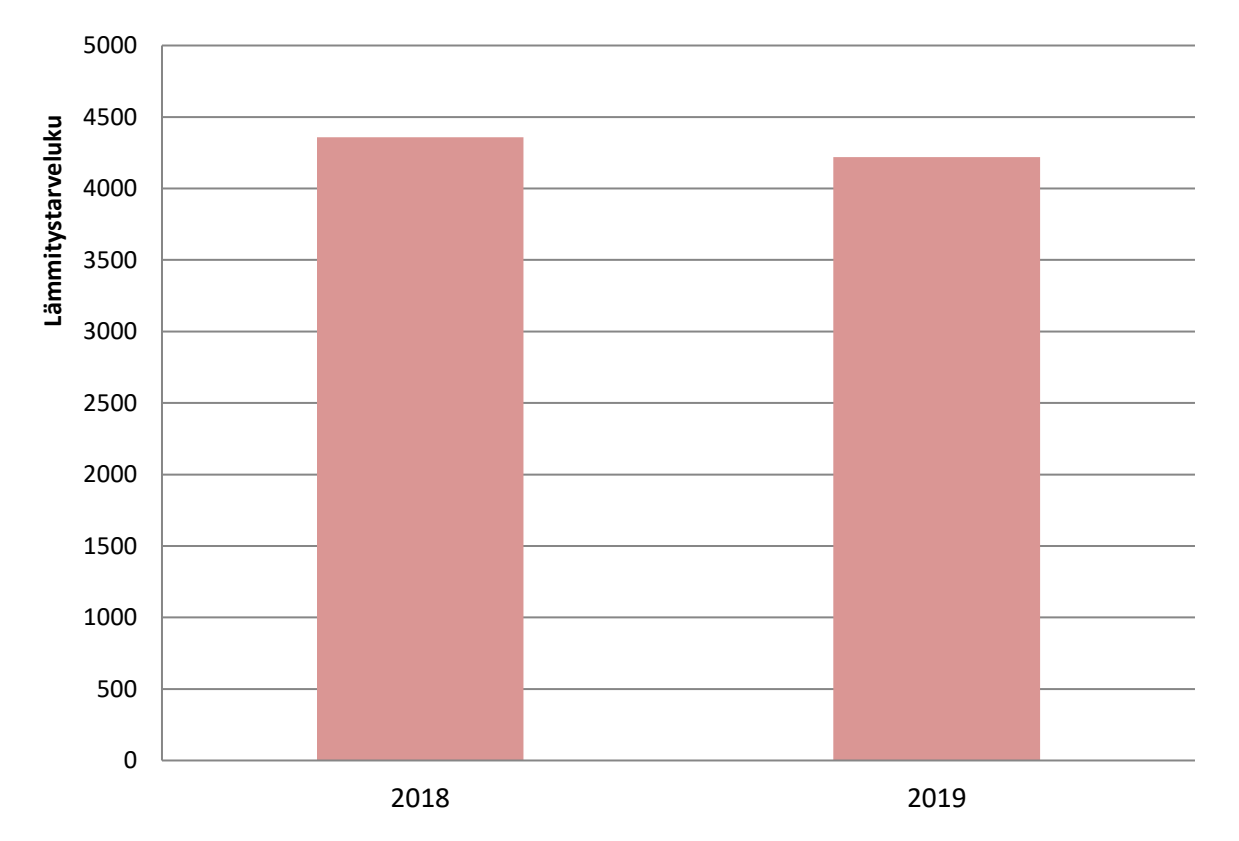
Kuva 4. Juvan lämmitystarveluvut vuosina 2018–2019.
