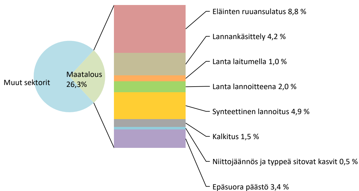
Kuva 9. Maatalouden päästöjen osuus kokonaispäästöistä (ilman teollisuutta) Juvalla vuonna 2018 ja sektorin jakautuminen eri päästölähteisiin.
