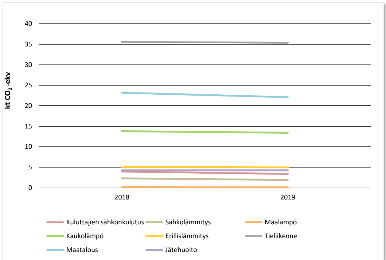
Kuva 16. Sektorikohtaisten päästöjen kehitys Juvalla vuosina 2018–2019. Vuoden 2019 tiedot perustuvat osittain ennakkotietoihin.
