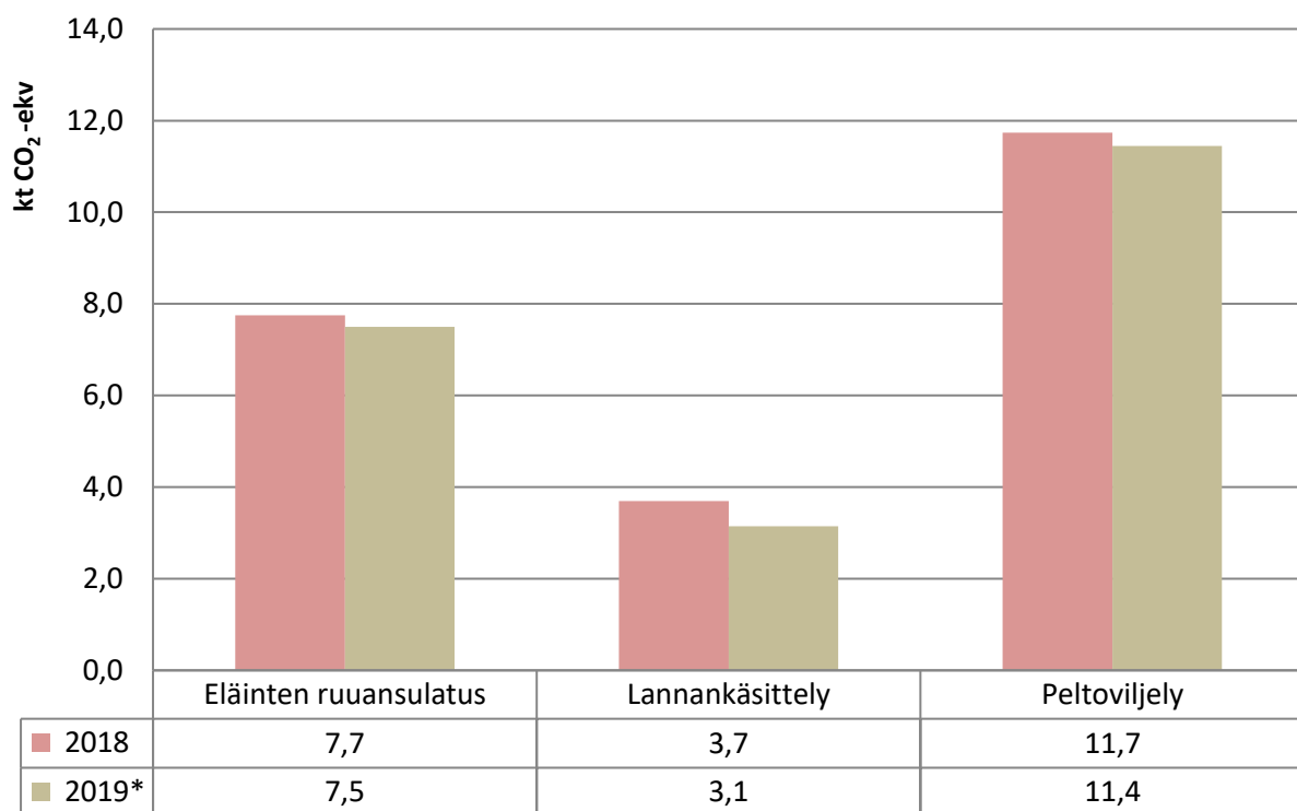
Kuva 10. Maatalouden päästöjen kehitys Juvalla vuosina 2018–2019 jaettuna eläinten ruuansulatuksen, lannankäsittelyn ja peltoviljelyn päästöihin.
