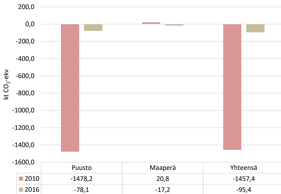
Kuva 26. Puuston ja maaperän kasvihuonekaasujen päästöt ja nielut Juvalla vuosina 2010 ja 2016.
