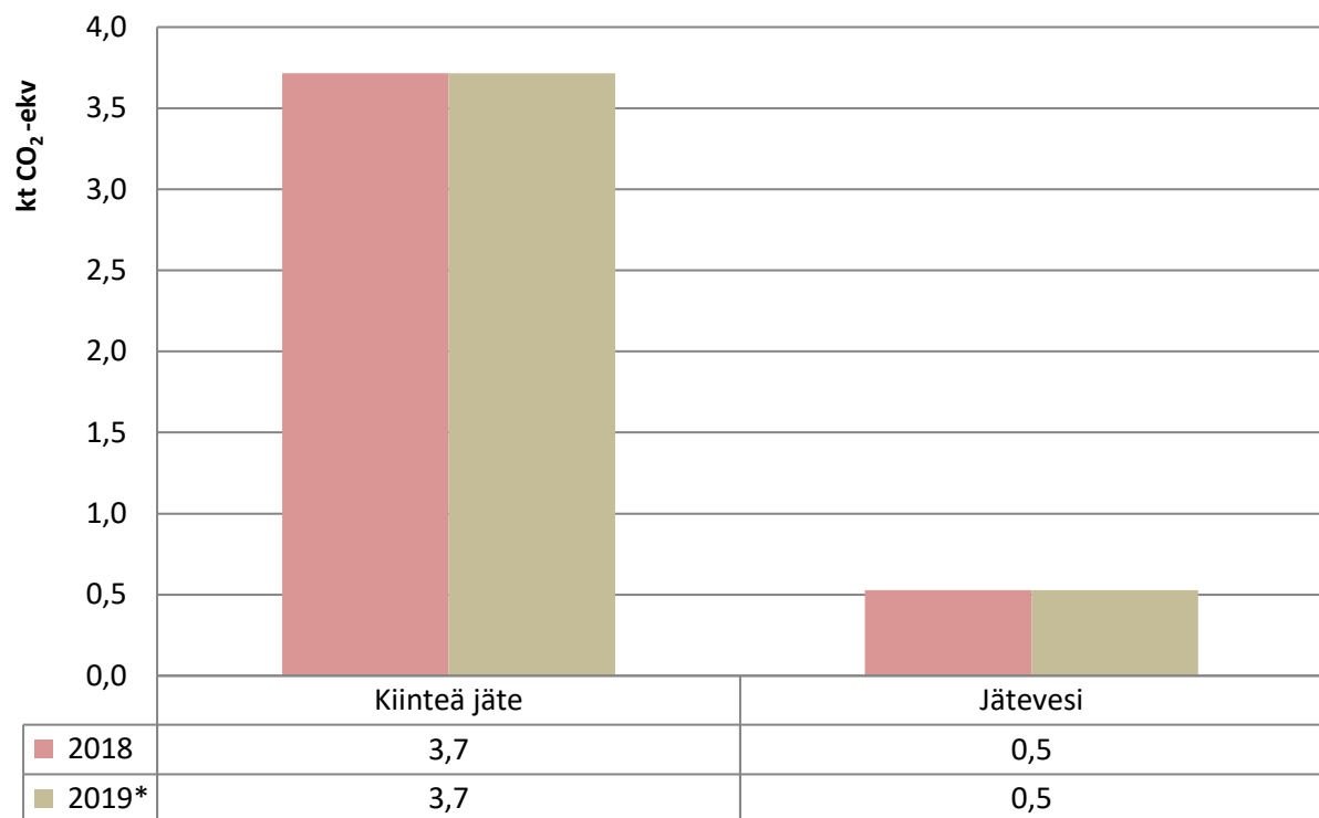
Kuva 12. Jätehuollon päästöjen kehitys Juvalla vuosina 2018–2019. Vuoden 2019 ennakkotietona on vuoden 2018 tieto.
