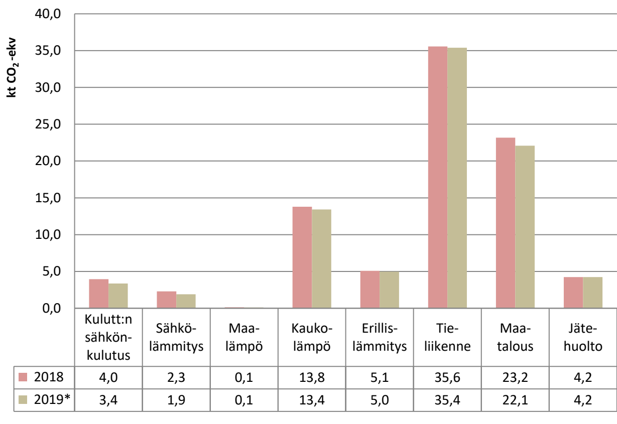
Kuva 15. Päästöt sektoreittain Juvalla vuosina 2018–2019 ilman teollisuutta. Vuoden 2019 tieto on ennakkotieto.
