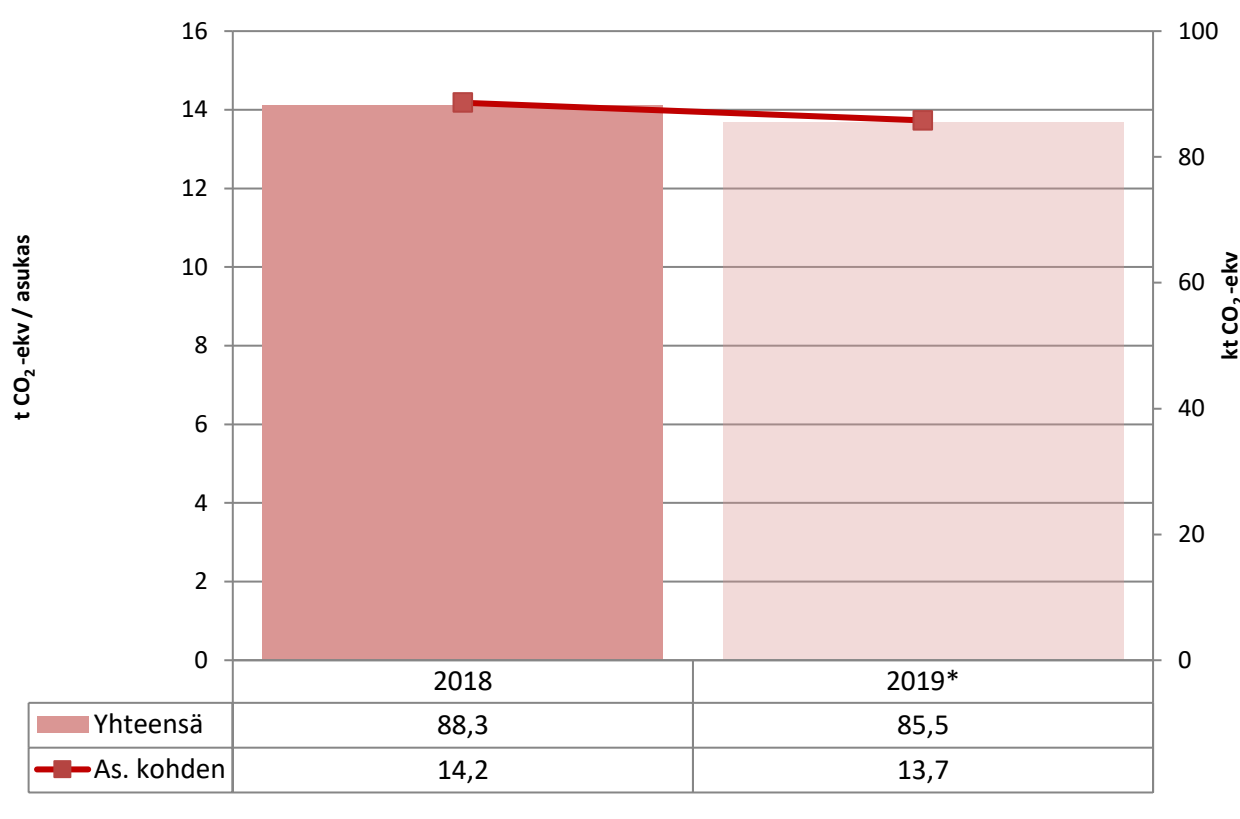
Kuva 17. Päästöt yhteensä ja asukasta kohden Juvalla vuosina 2018–2019 ilman teollisuutta. Vuoden 2019 tieto on ennakkotieto.
