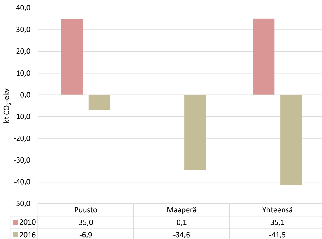
Kuva 26. Puuston ja maaperän kasvihuonekaasujen päästöt ja nielut Mäntyharjulla vuosina 2010 ja 2016.
