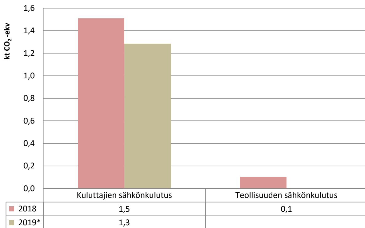
Kuva 3. Kuluttajien ja teollisuuden sähkönkulutuksen päästöjen kehitys Pertunmaalla vuosina 2018–2019. Vuoden 2019 tieto on ennakkotieto. Sitä ei ole esitetty teollisuuden sähkönkulutukselle.
