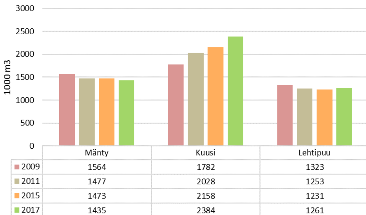
Kuva 24. Puuston tilavuus puulajeittain Pertunmaalla 2009–2017 (Metla, Luke/VMI).
