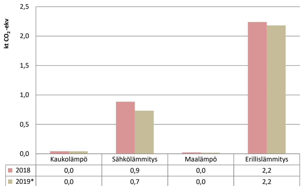
Kuva 6. Rakennusten lämmityksen päästöjen kehitys Pertunmaalla vuosina 2018–2019. Vuoden 2019 tieto on ennakkotieto.
