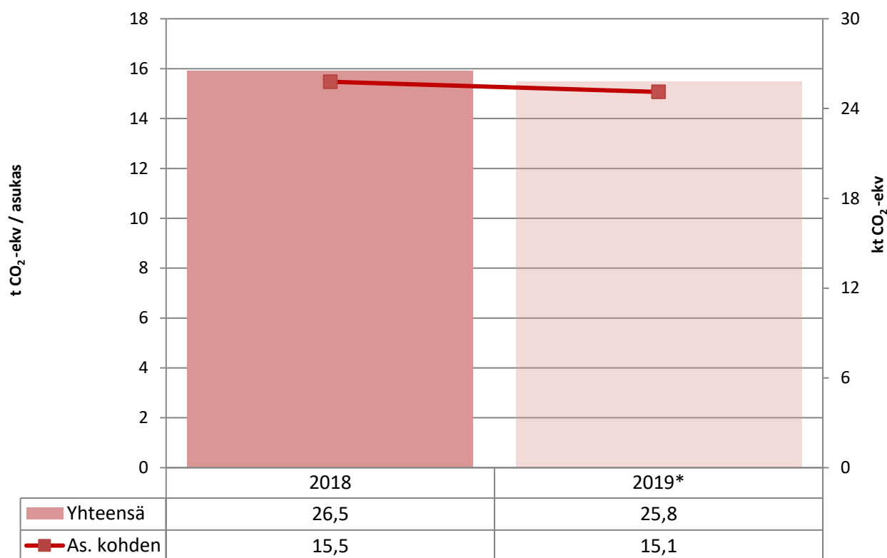
Kuva 17. Päästöt yhteensä ja asukasta kohden Pertunmaalla vuosina 2018–2019 ilman teollisuutta. Vuoden 2019 tieto on ennakkotieto.
