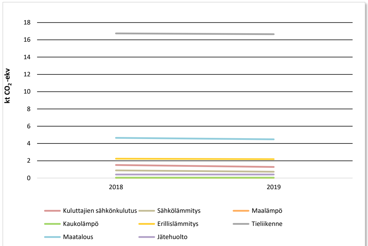
Kuva 16. Sektorikohtaisten päästöjen kehitys Pertunmaalla vuosina 2018–2019. Vuoden 2019 tiedot perustuvat osittain ennakkotietoihin.
