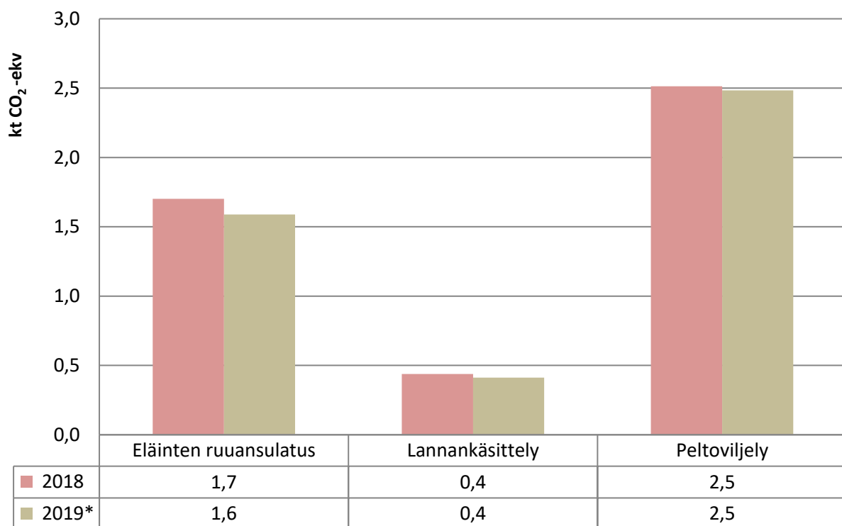
Kuva 10. Maatalouden päästöjen kehitys Pertunmaalla vuosina 2018–2019 jaettuna eläinten ruuansulatuksen, lannankäsittelyn ja peltoviljelyn päästöihin.
