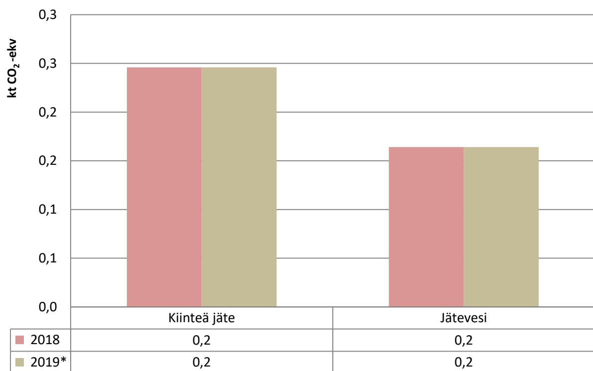
Kuva 12. Jätehuollon päästöjen kehitys Pertunmaalla vuosina 2018–2019. Vuoden 2019 ennakkotietona on vuoden 2018 tieto.
