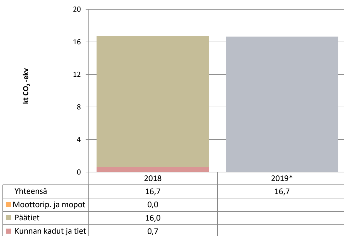
Kuva 8. Tieliikenteen päästöt Pertunmaalla vuosina 2018–2019. Vuoden 2019 tieto on ennakkotieto.
