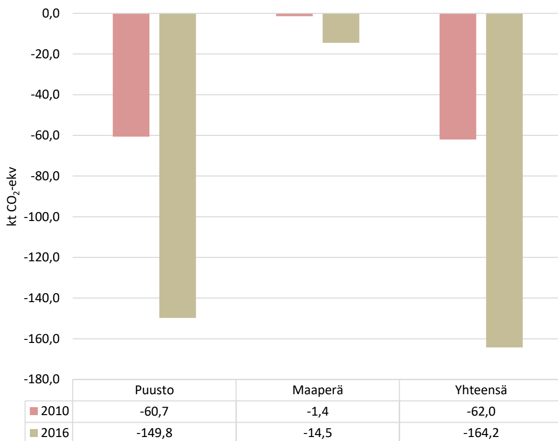
Kuva 26. Puuston ja maaperän kasvihuonekaasujen päästöt ja nielut Pertunmaalla vuosina 2010 ja 2016.
