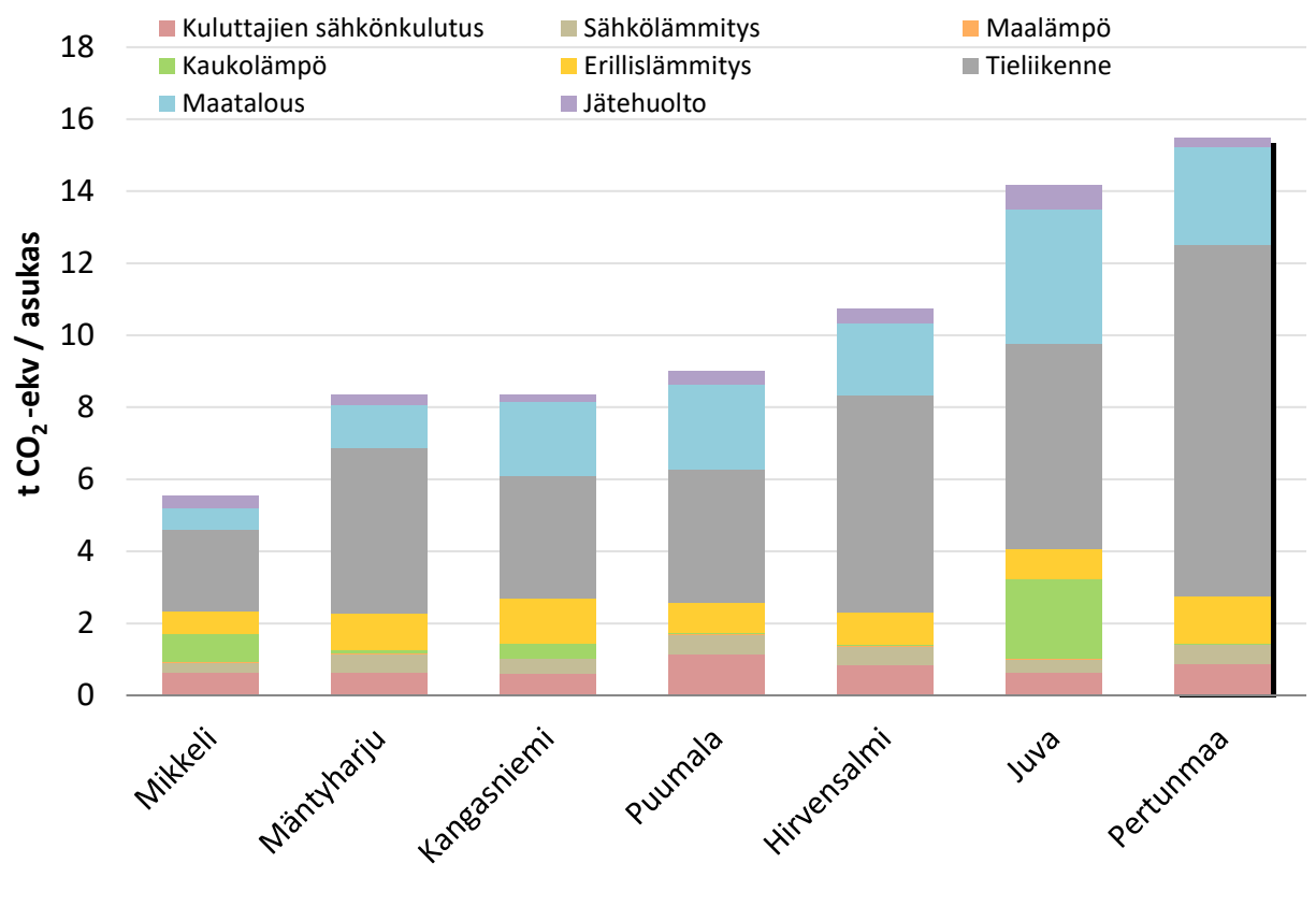
Kuva 19. CO2-raportissa mukana olevien Etelä-Savon kuntien asukaskohtaiset päästöt vuonna 2018 ilman teollisuutta.
