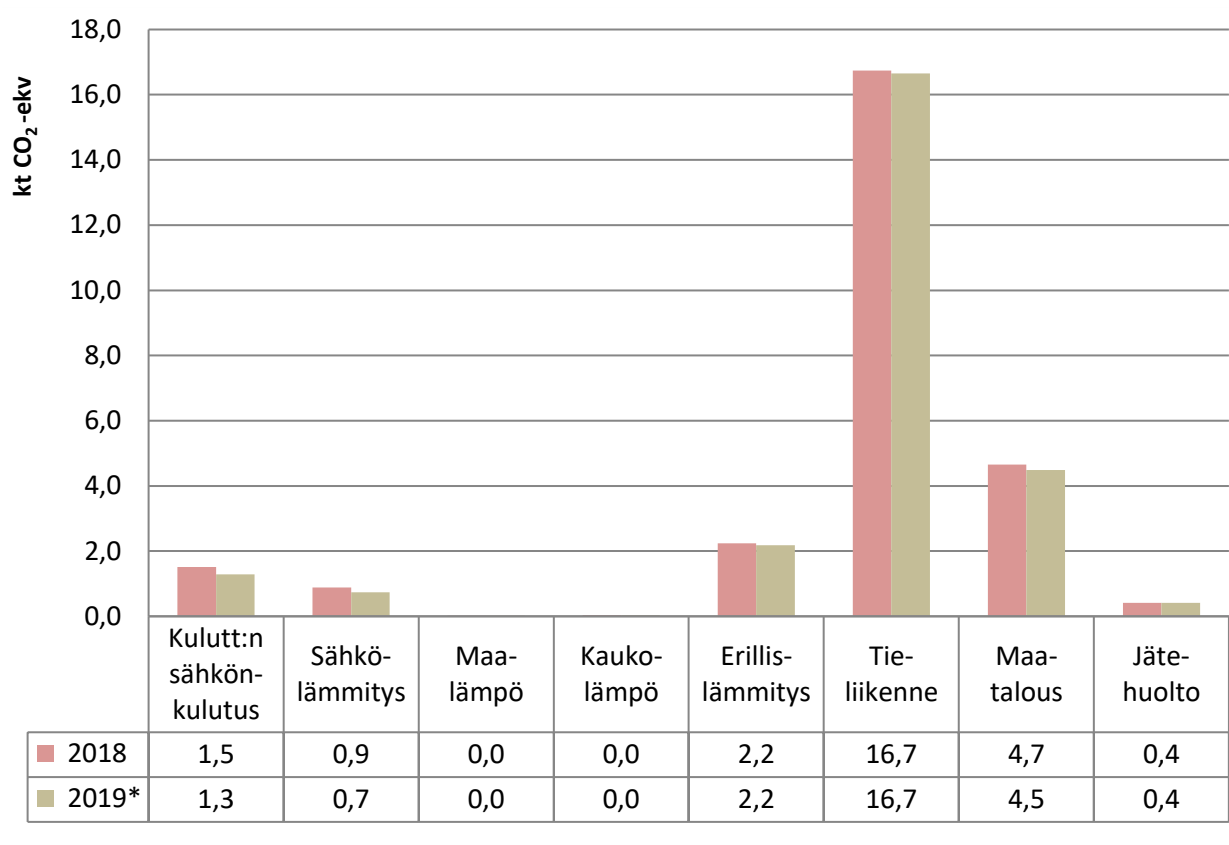
Kuva 15. Päästöt sektoreittain Pertunmaalla vuosina 2018–2019 ilman teollisuutta. Vuoden 2019 tieto on ennakkotieto.
