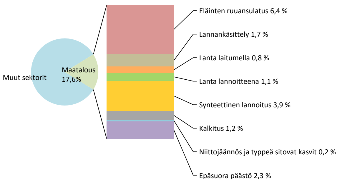
Kuva 9. Maatalouden päästöjen osuus kokonaispäästöistä (ilman teollisuutta) Pertunmaalla vuonna 2018 ja sektorin jakautuminen eri päästölähteisiin.
