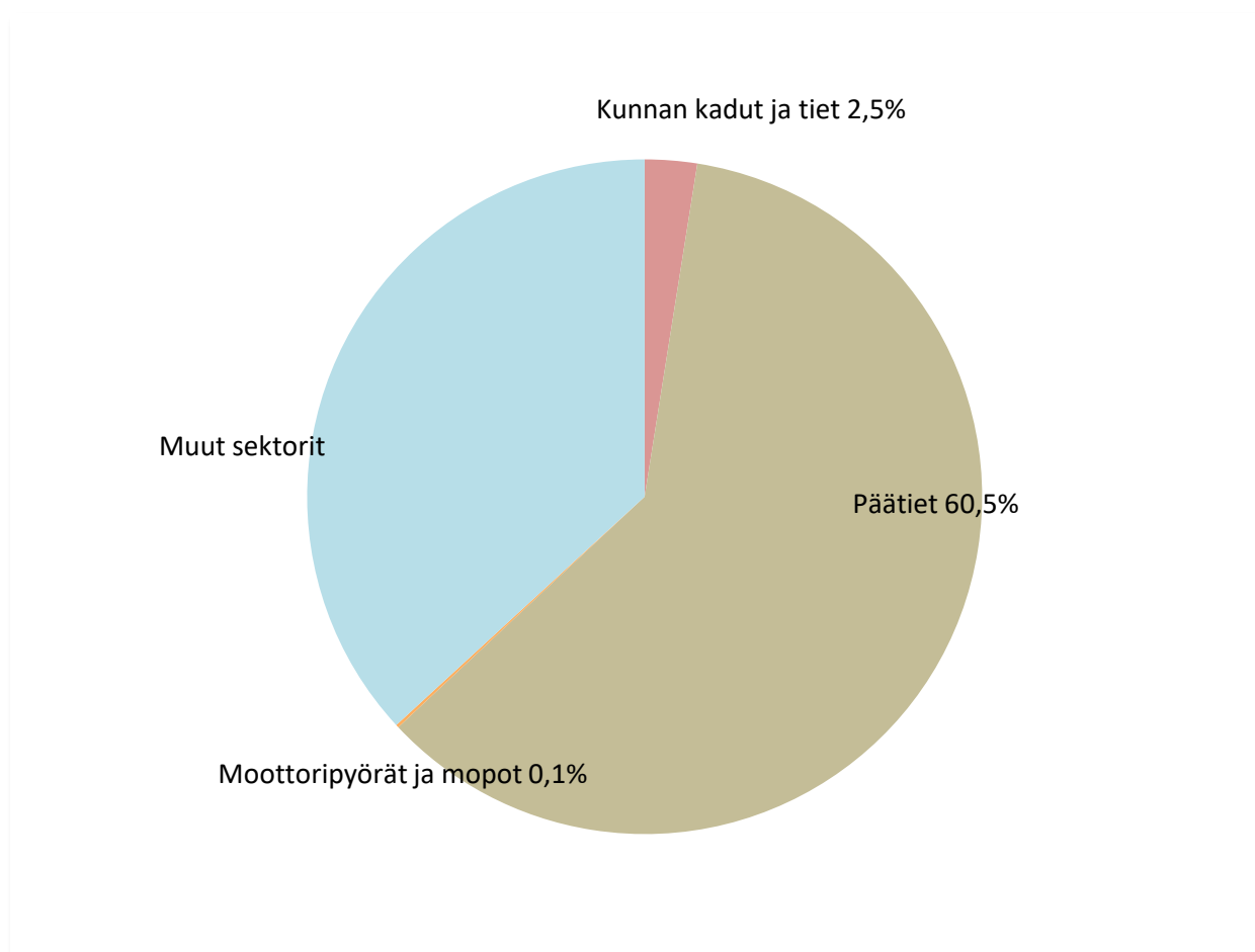
Kuva 7. Tieliikenteen päästöjen osuus kokonaispäästöistä (ilman teollisuutta) Pertunmaalla vuonna 2018 ja sektorin jakautuminen eri päästölähteisiin.
