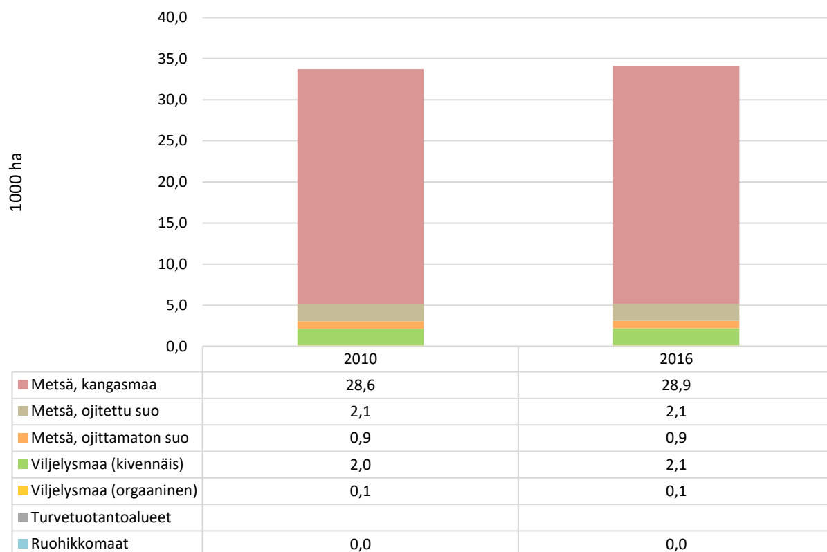
Kuva 25. Maankäyttösektorin laskennassa mukana olevien maankäyttömuotojen pinta-alat Pertunmaalla vuosina 2010 ja 2016 (Metla, Luke/VMI, Maaseutuvirasto/Ruokavirasto, ELY-keskus).
