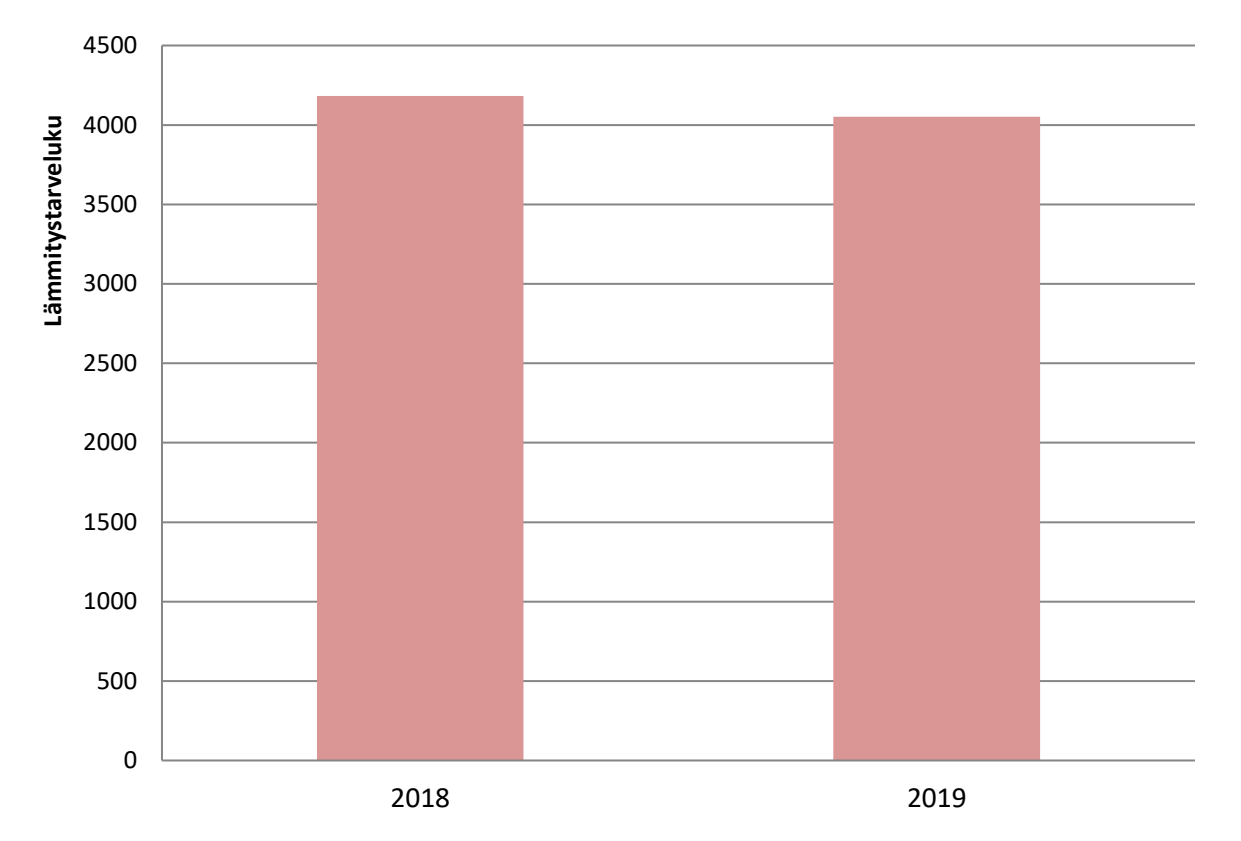
Kuva 4. Pertunmaan lämmitystarveluvut vuosina 2018–2019.
