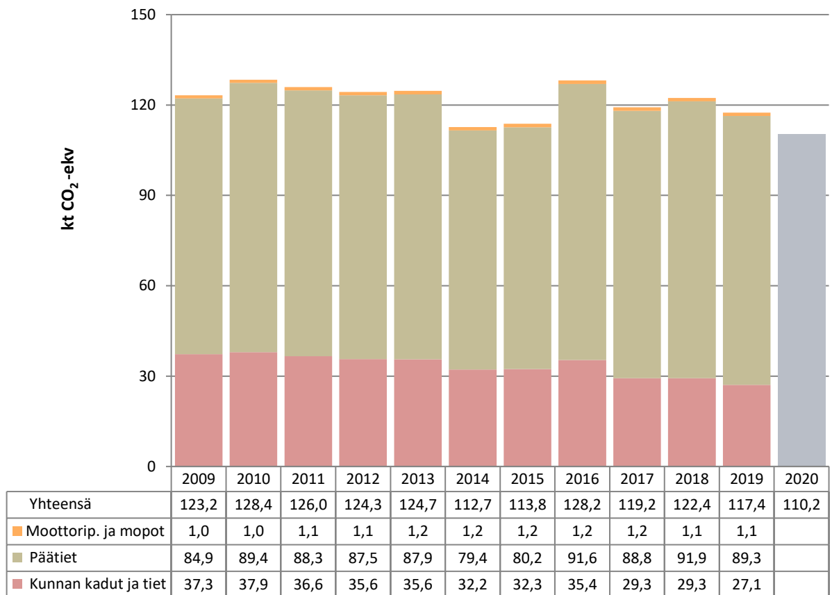
Kuva 8. Tieliikenteen päästöt Mikkelissä vuosina 2009–2020. Vuoden 2020 tieto on ennakkotieto, joka perustuu liikennemäärien muutoksiin kunnan alueella.
