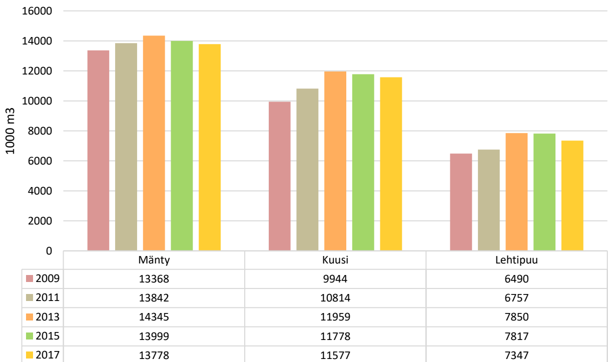
Kuva 20. Puuston tilavuus puulajeittain Mikkelissä 2009–2017 (Metla, Luke/VMI).
