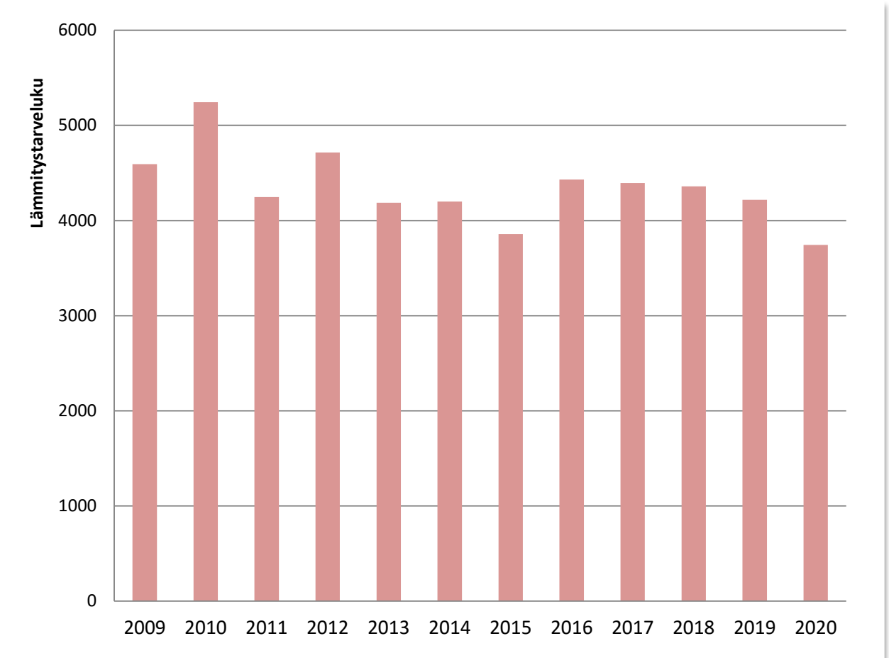
Kuva 4. Mikkelin lämmitystarveluvut vuosina 2009–2020.
