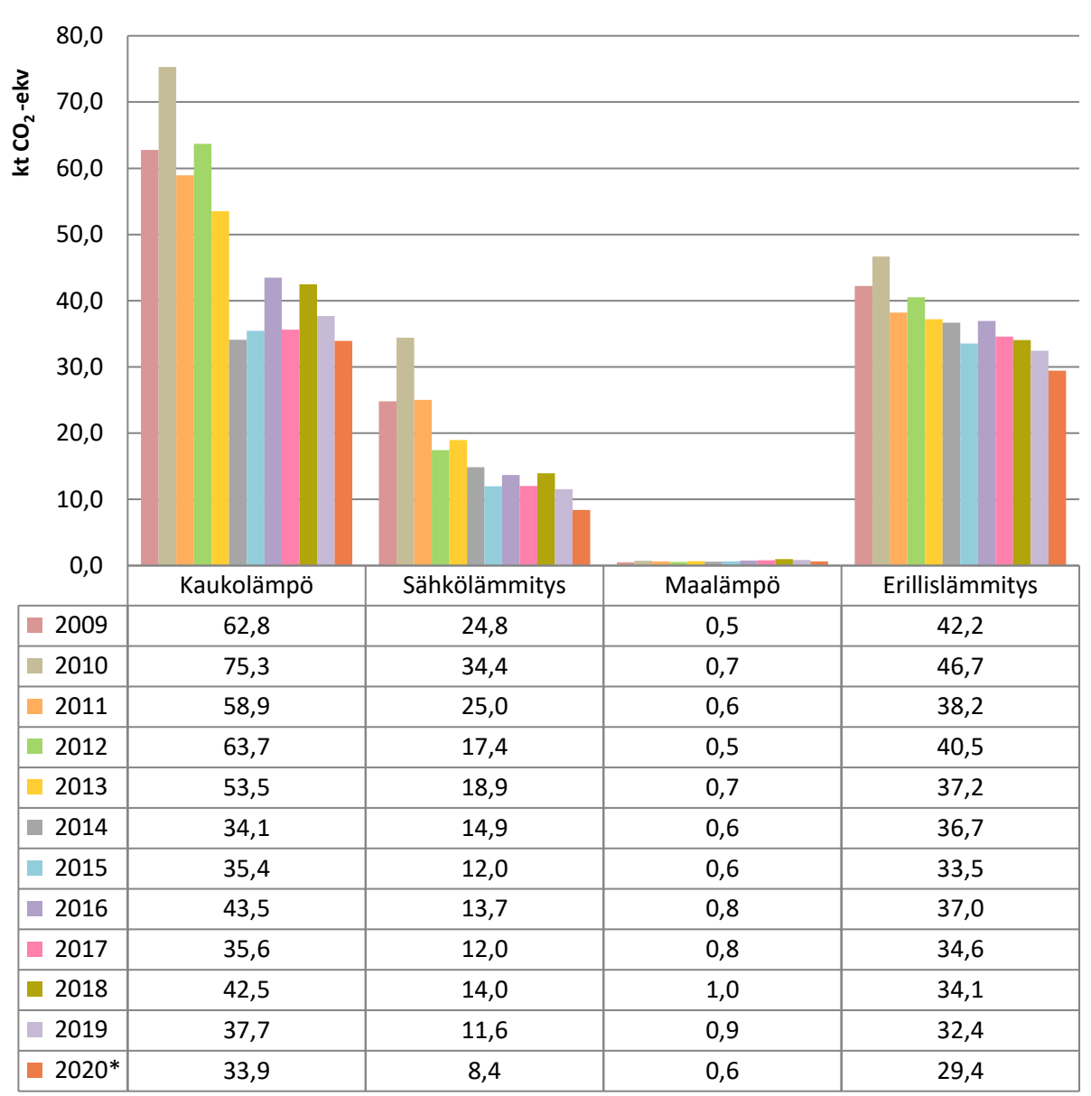
Kuva 6. Rakennusten lämmityksen päästöjen kehitys Mikkelissä vuosina 2009–2020. Vuoden 2020 tieto on ennakkotieto.
