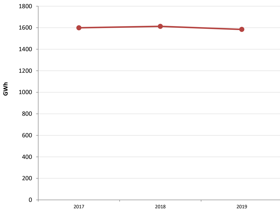
Kuva 24. Energian loppukulutuksen kehitys Mikkelissä vuosina 2017–2019 ilman teollisuutta. Energian loppukulutus ei sisällä lämpöpumppujen tuottamaa uusiutuvaa energiaa, mutta sisältää niiden käyttämän sähkön.
