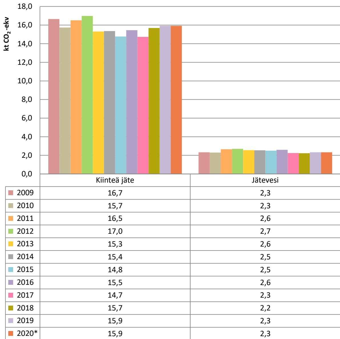
Kuva 12. Jätehuollon päästöjen kehitys Mikkelissä vuosina 2009–2020. Vuoden 2020 ennakkotietona on vuoden 2019 tieto.
