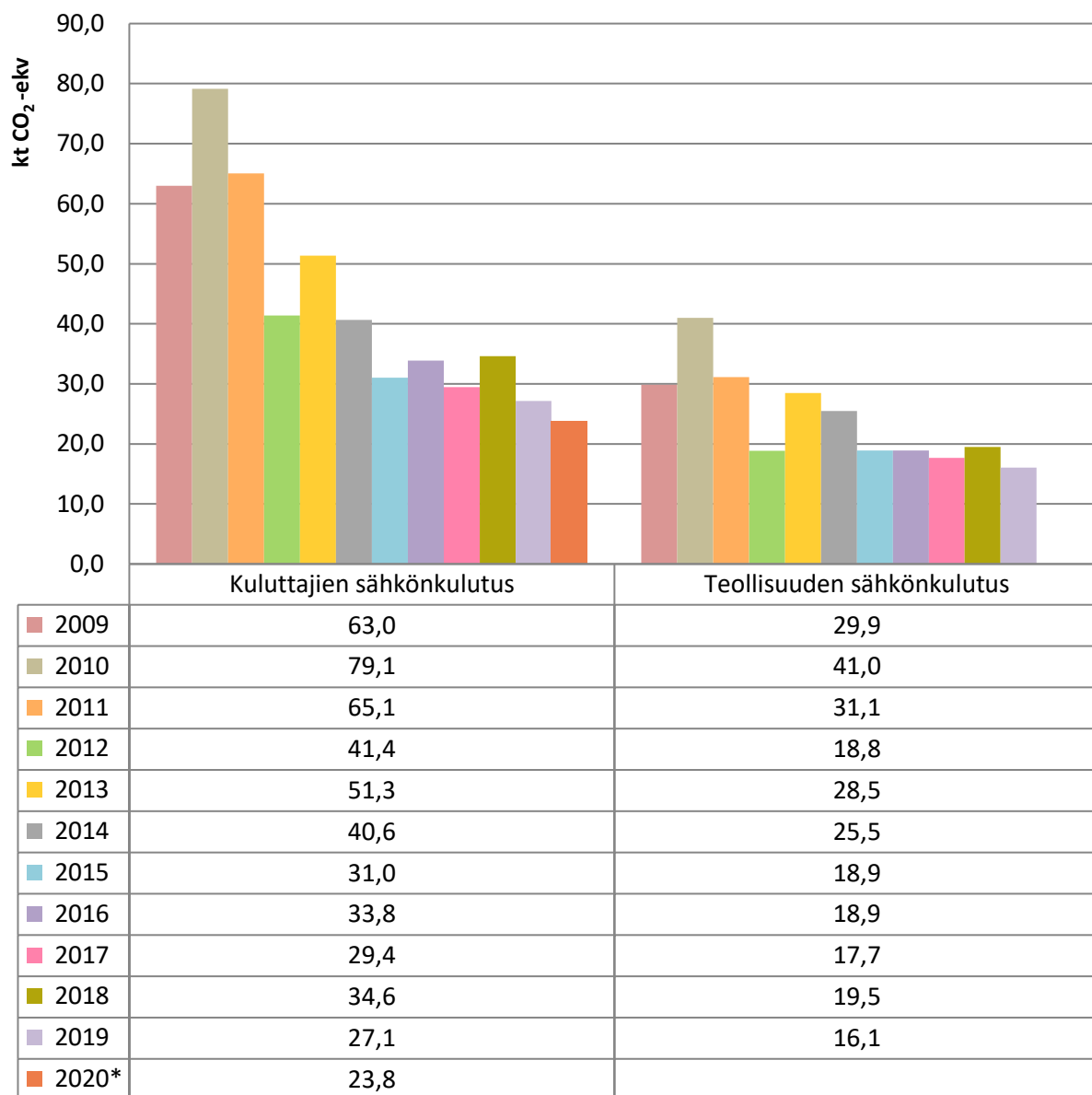
Kuva 3. Kuluttajien ja teollisuuden sähkönkulutuksen päästöjen kehitys Mikkelissä vuosina 2009–2020. Vuoden 2020 tieto on ennakkotieto. Sitä ei ole esitetty teollisuuden sähkönkulutukselle.
