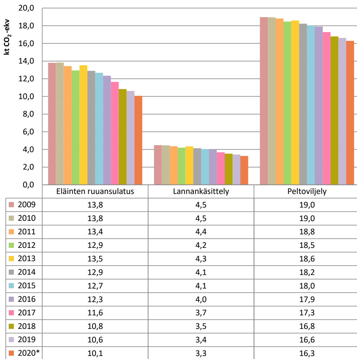
Kuva 10. Maatalouden päästöjen kehitys Mikkelissä vuosina 2009–2020 jaettuna eläinten ruuansulatuksen, lannankäsittelyn ja peltoviljelyn päästöihin.
