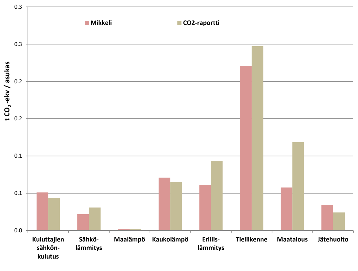
Kuva 17. Asukaskohtaisten päästöjen vertailu keskimääräiseen CO 2 -raportin kuntaan vuonna 2019.
