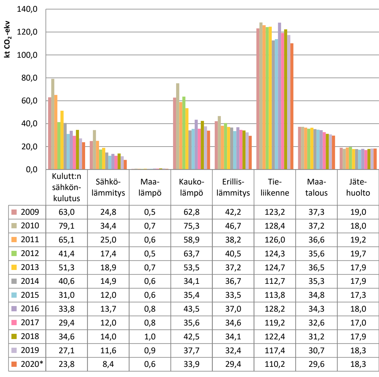
Kuva 14. Päästöt sektoreittain Mikkelissä vuosina 2009–2020 ilman teollisuutta. Vuoden 2020 tieto on ennakkotieto.
