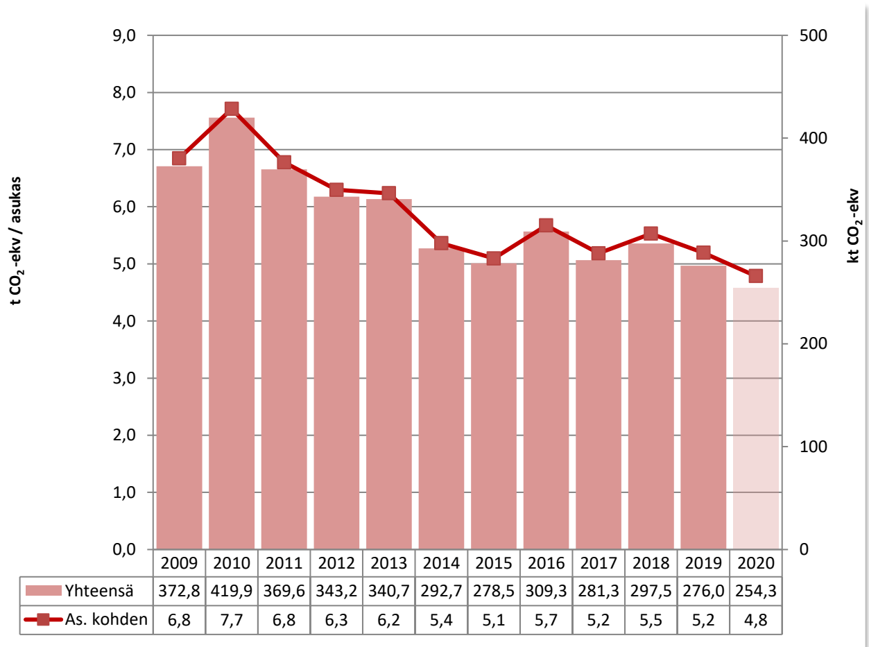
Kuva 16. Päästöt yhteensä ja asukasta kohden Mikkelissä vuosina 2009–2020 ilman teollisuutta. Vuoden 2020 tieto on ennakkotieto.
