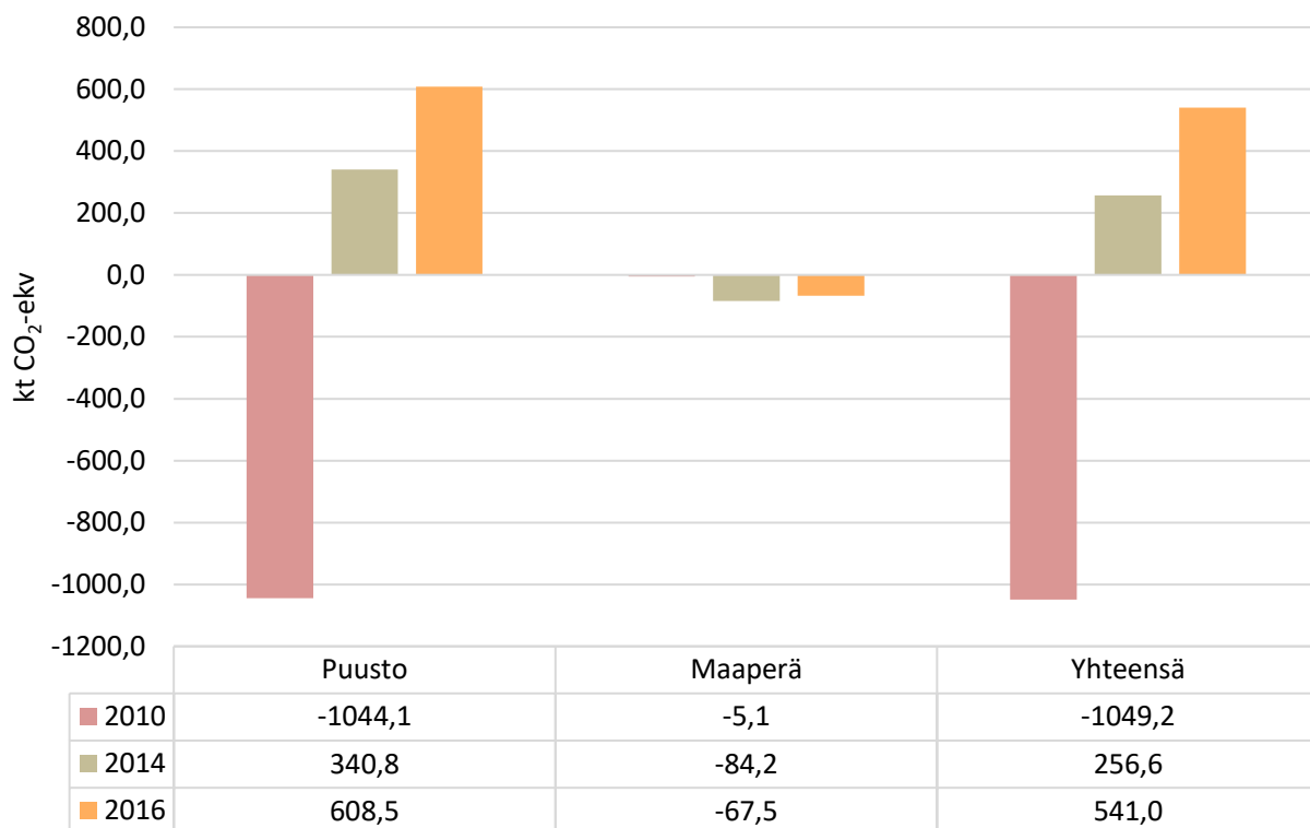
Kuva 22. Puuston ja maaperän kasvihuonekaasujen päästöt ja nielut Mikkelissä vuosina 2010, 2014 ja 2016.
