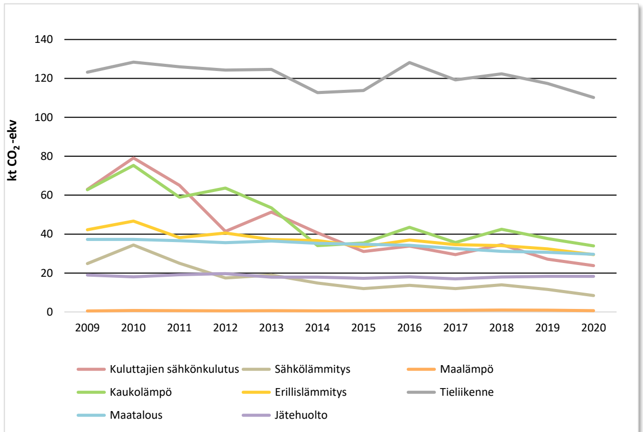
Kuva 15. Sektorikohtaisten päästöjen kehitys Mikkelissä vuosina 2009–2020. Vuoden 2020 tiedot perustuvat osittain ennakkotietoihin.
