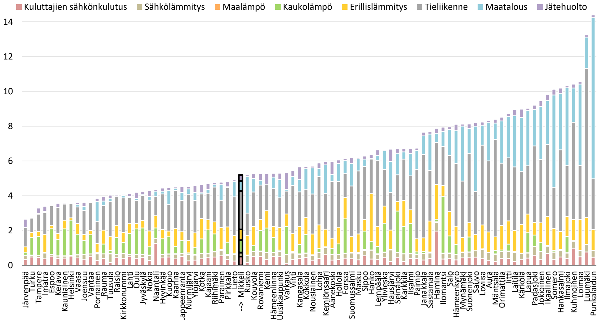
Kokonaispäästöt kaikissa CO2-raportin kunnissa vuonna 2019 ilman teollisuutta (t CO 2 -ekv/asukas)
