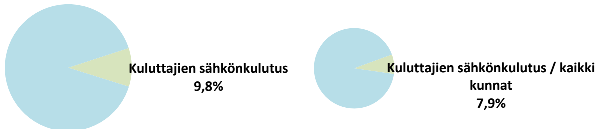
Kuva 2. Kuluttajien sähkönkulutuksen päästöjen osuus kokonaispäästöistä (ilman teollisuutta) Mikkelissä ja CO2-raportin kunnissa keskimäärin vuonna 2019.
