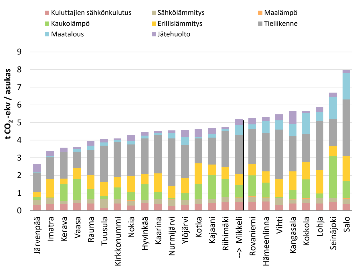
Kuva 18. CO 2 -raportissa mukana olevien 25 000–70 000 asukkaan kuntien asukaskohtaiset päästöt vuonna 2019 ilman teollisuutta.
