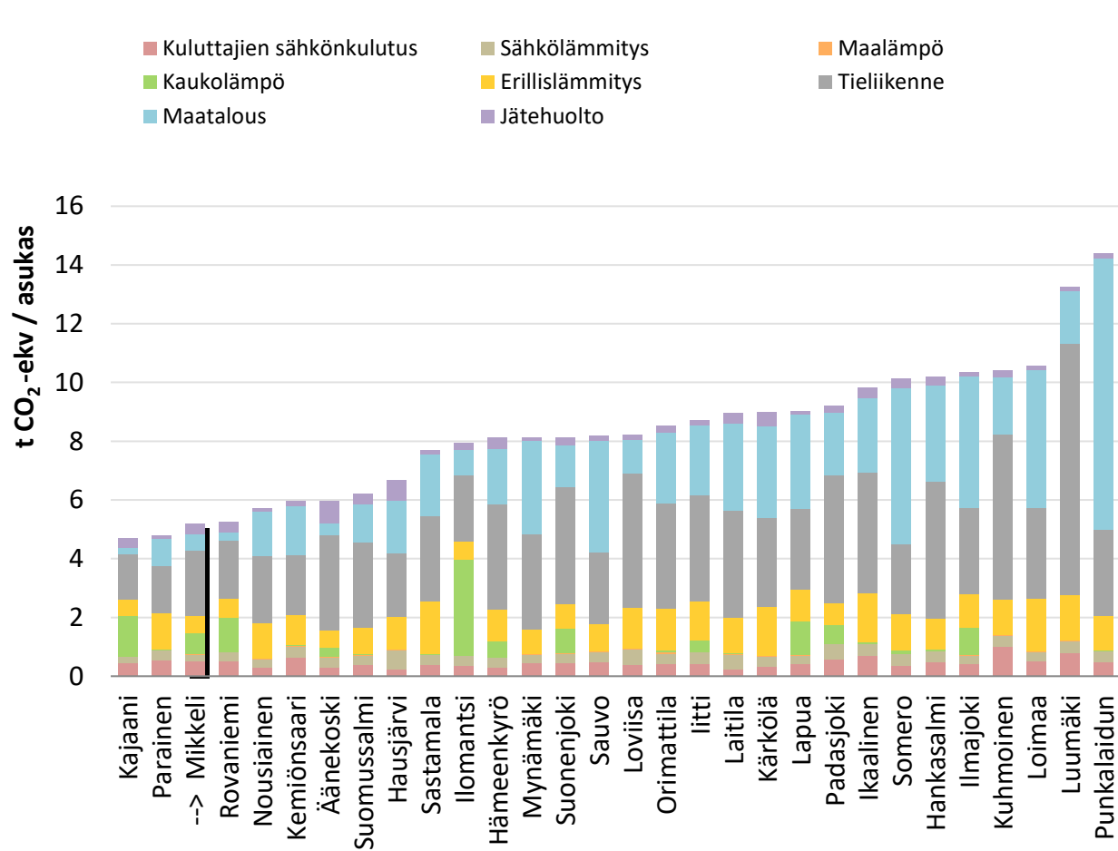
Kuva 19. Asukaskohtaisten päästöjen vertailu (ilman teollisuutta) vuonna 2019 sellaisissa CO2-raportin kunnissa, joissa on alle 25 asukasta maaneliökilometrillä.
