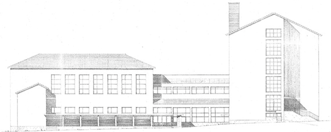
Julkisivu etelään. (Mikkelin rakennusvalvonta)
