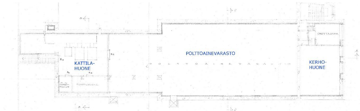
Kellarikerros. (Pohjapiirros Mikkelin rakennusvalvonta)
