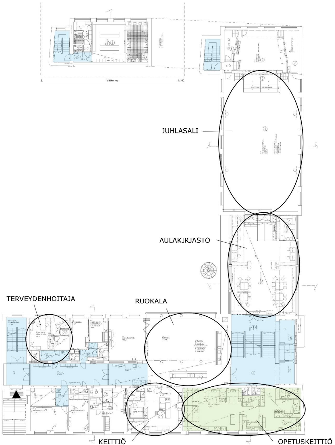
Urheilupuiston koulun ensimmäinen kerros.
