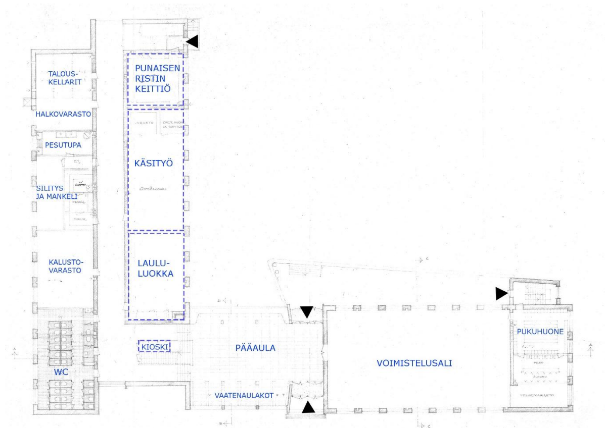
Pohjakerros. (Pohjapiirros Mikkelin rakennusvalvonta)
