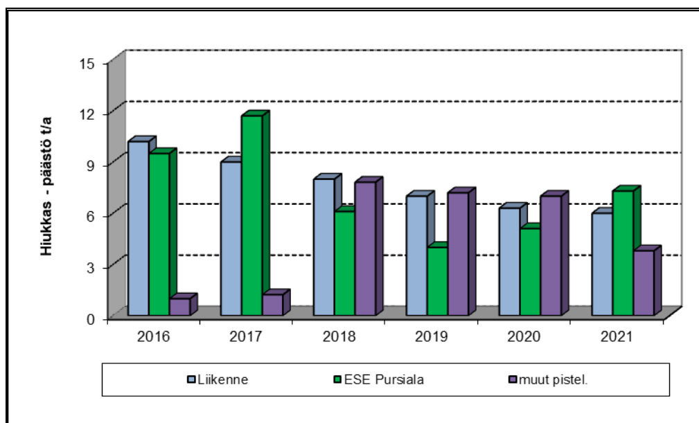
Kuva 2-2 Mikkelin kaupunkiseudun ilmoitusvelvollisten laitosten ja liikenteen hiukkaspäästöt ilmaan vuosina 2016-2021.
