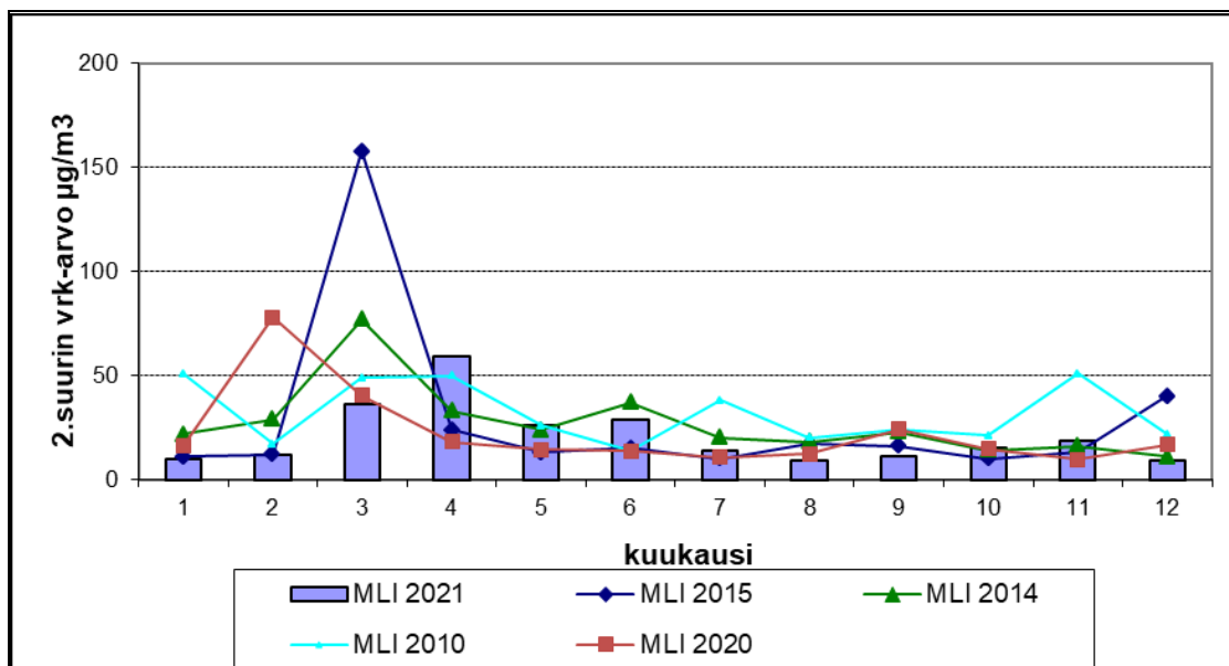
Kuva 7-1 Hengitettävän pölyn ohjearvoon verrattava kuukauden toiseksi suurin vuorokausiarvo Mikkelissä Porrassalmenkadun mittausaseman mittauspisteellä vuonna 2021 (sekä aiemmat mittaukset 2010-2015; 2020). Ohjearvo on 70 \mu\text{g}/\text{m}^3 .
