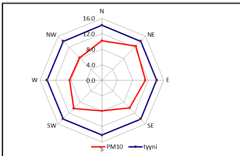
Kuva 7-5 Hengitettävän pölyn tuntiarvojen keskiarvopitoisuudet eri tuulen suunnilla Mikkelin Porrassalmenkadun mittausasemalla vuonna 2021. Tyyneksi lasketaan tuulen nopeus alle 0,5 m/s.
