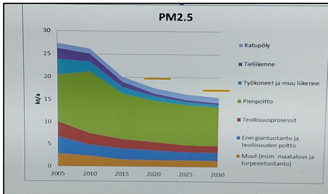
Kuva 2-4 Hiukkaspäästöjen (tonnia/vuosi) kehitys vuosina 2005-2030 Suomessa vuoden 2017 tietojen mukaan (Sirpa Salo-Asikainen 2019).
