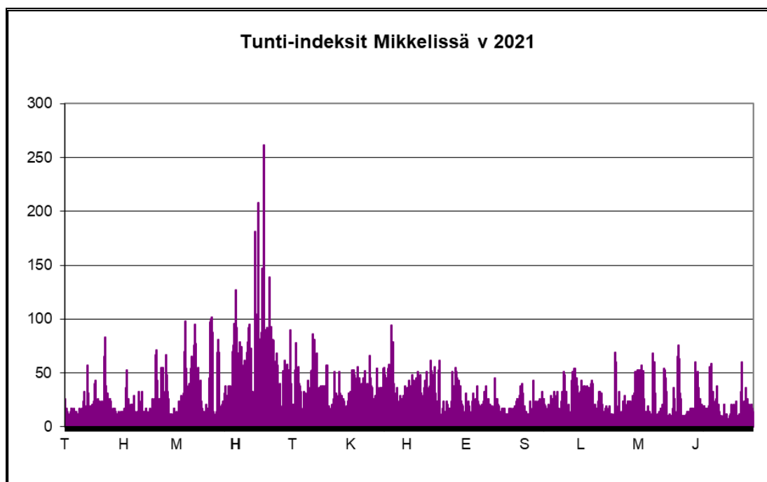
Kuva 9-2 Ilmanlaatuindeksit Mikkelin Porrassalmenkadun mittausasemalla vuonna 2021.
