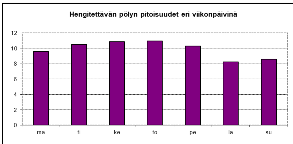
Kuva 7-4 Hengitettävän pölyn pitoisuudet ( \mu\text{g}/\text{m}^3 ) eri viikonpäivinä Mikkelin Porrassalmenkadun mittausasemalla vuonna 2021.
