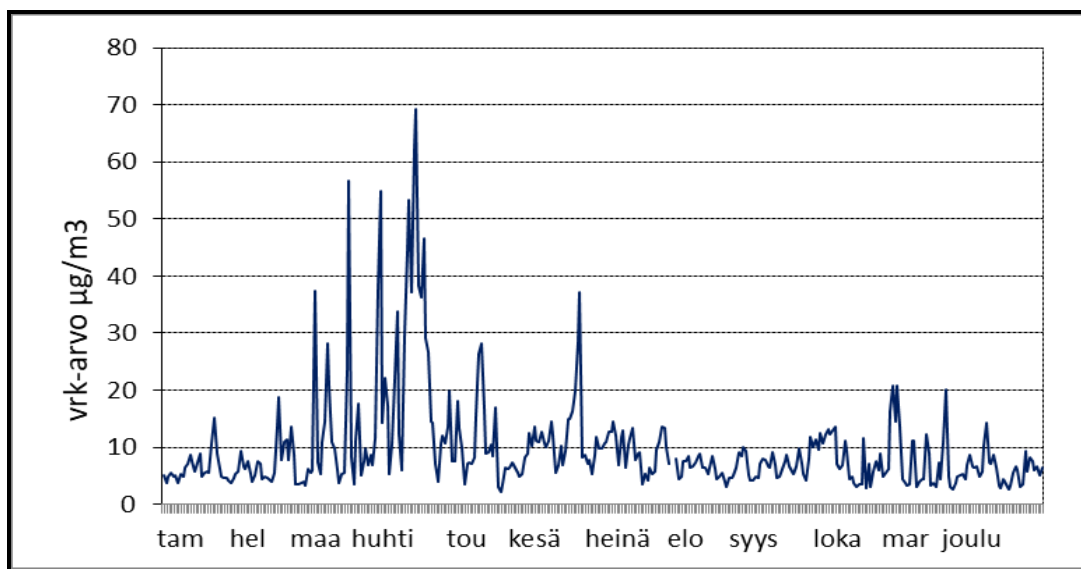
Kuva 7-2 Hengitettävän pölyn vuorokausiarvot Mikkelin Porrassalmenkadun mittausaseman mittauspisteellä vuonna 2021 (pitoisuudet laskettu vallitseviin olosuhteisiin).
