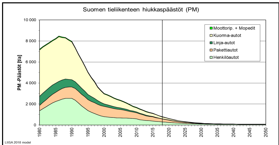
Kuva 2-3 Tieliikenteen hiukkaspäästöjen (tonnia/vuosi) kehitys vuosina 1980-2050 Suomessa vuoden 2019 tietojen mukaan (Liisa 2019).
