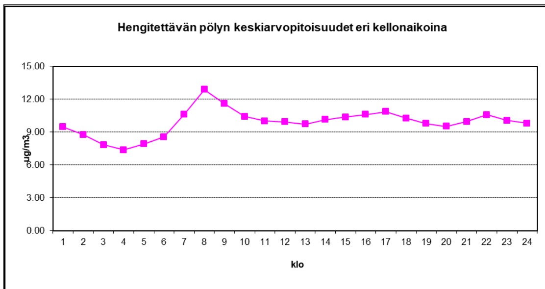
Kuva 7-3 Hengitettävän pölyn pitoisuudet ( \mu\text{g}/\text{m}^3 ) eri kellonaikoina Mikkelin Porrassalmenkadun mittausasemalla vuonna 2021.
