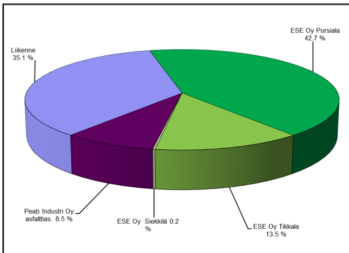
Kuva 2-1 Mikkelin kaupunkiseudun ilmoitusvelvollisten laitosten ja liikenteen hiukkaspäästöjakauma (%) v 2021.
