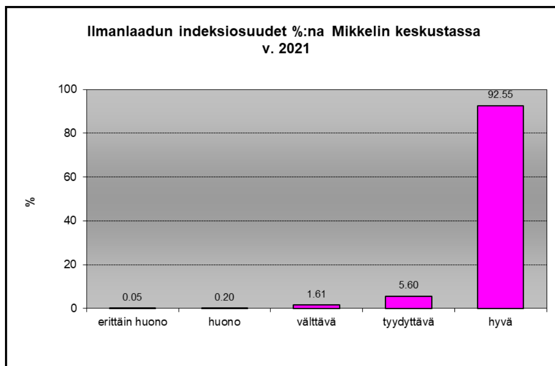
Kuva 9-1 Ilmanlaatuindeksin eri luokkien %-osuudet Mikkelin Porrassalmenkadun mittausasemalla vuonna 2021.
