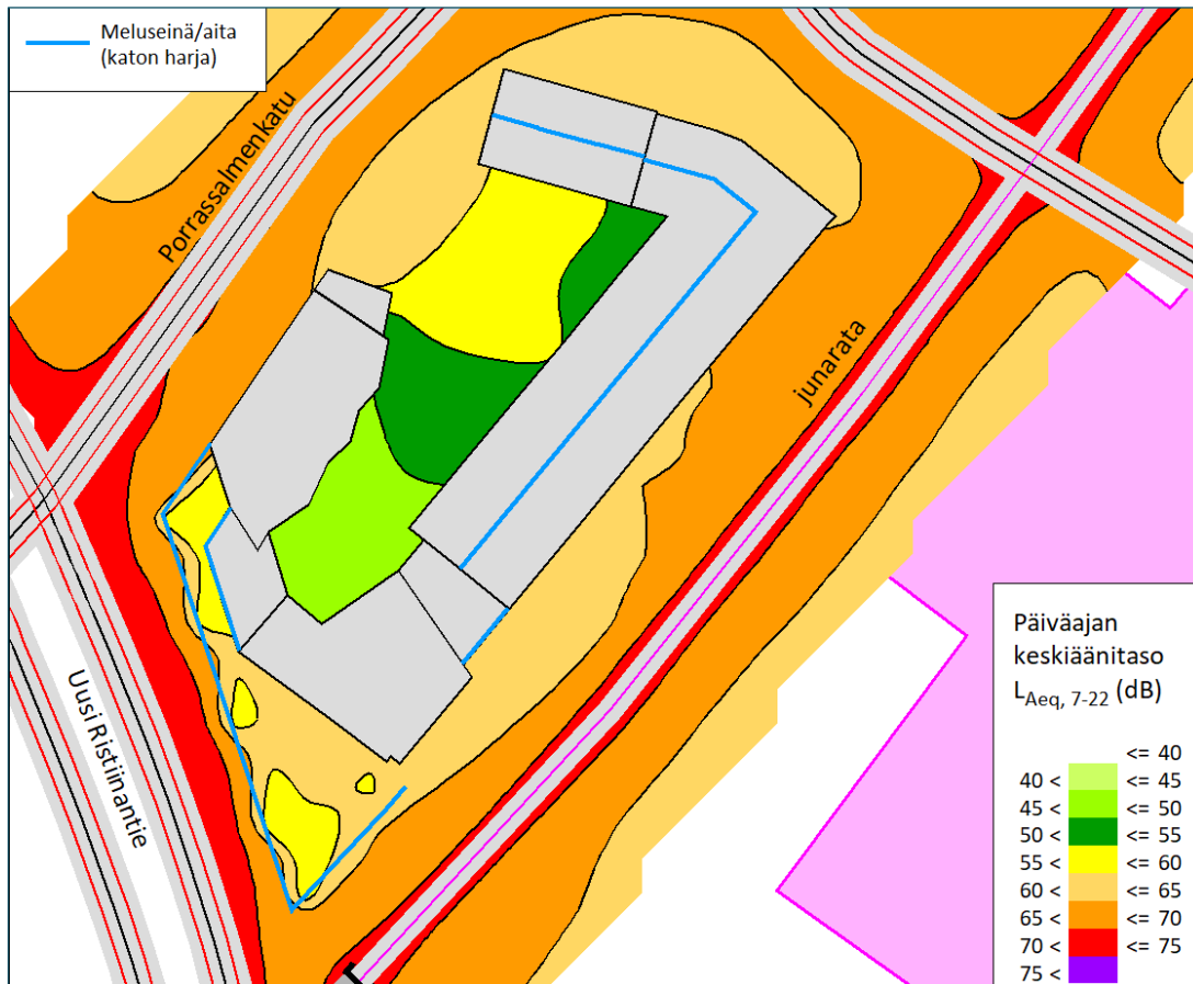
Kuvaote meluselvityksestä. Kuvassa päivääjan ennustettu keskiäänitaso, joka on laskettu vuoden 2040 liikenne-ennusteen sekä veturitallin puolelle rakentuvan hypermarketin aiheuttaman liikenteen perusteella.
