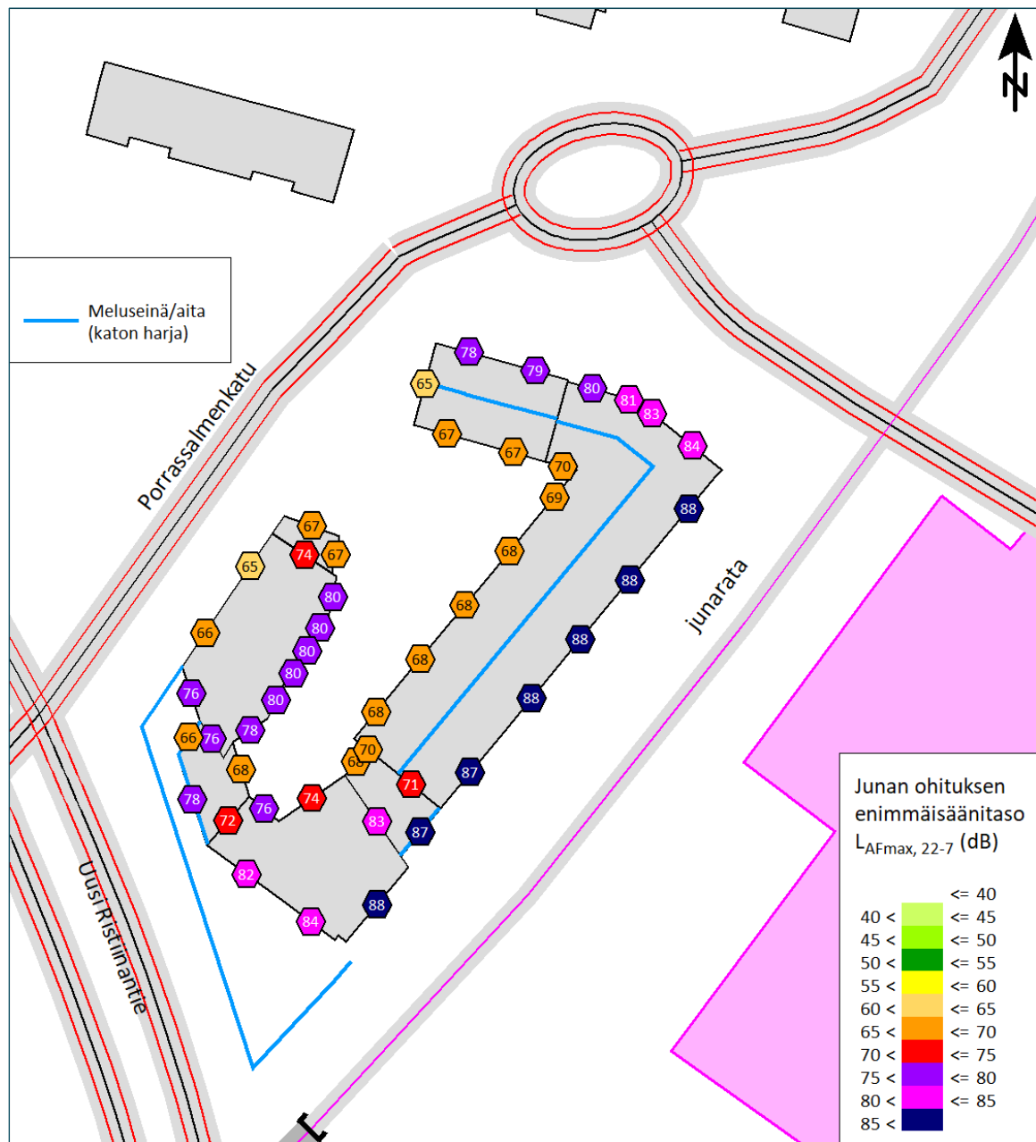
Kuva 7 Tavarajunan ohiajan enimmäisäänitaso yöllä.
