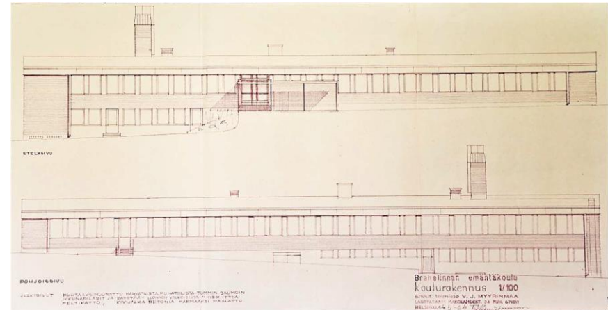
Kuva: Brahelinann emäntäkoulun julkisivupiirustukset./ Koulurakennus 1964. Arkkitehti V. J. Myyrinmaalla (1910-2007) oli oma arkkitehtitoimisto 1953–1969. Brahelinann emäntäkoulun hän suunnitteli aikana, jolloin hän toimi myös Rakennushallituksen toimistoarkkitehtina, vuonna 1966 hän siirtyi Kouluhallituksen yliarkkitehdiksi, josta virasta siirtyi eläkkeelle 1977.
