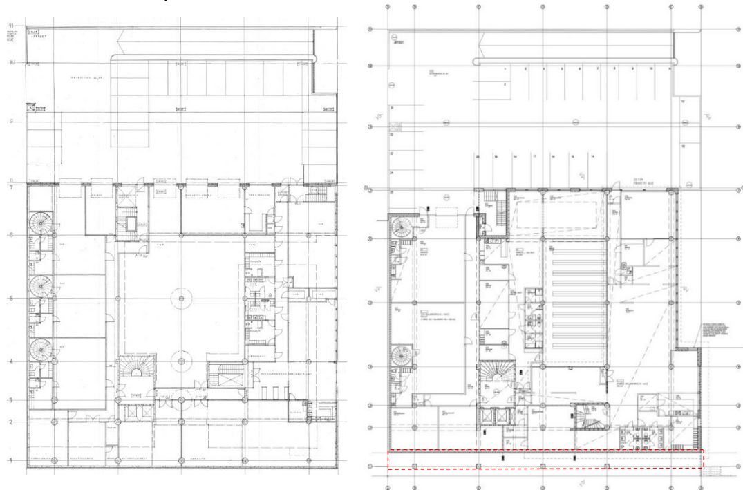
Kuva 11. (vas.) Yläkellarin pohjapiirustus, pääpiirustus, Arkkitetoimisto Eino Tuompo, Helsinki (1977 05 12). Kuva 12. (oik). Alakellarin nykytilanpohjapiirustus, Arkkitetoimisto Heikki Kirjalainen, 22.7.2009.
