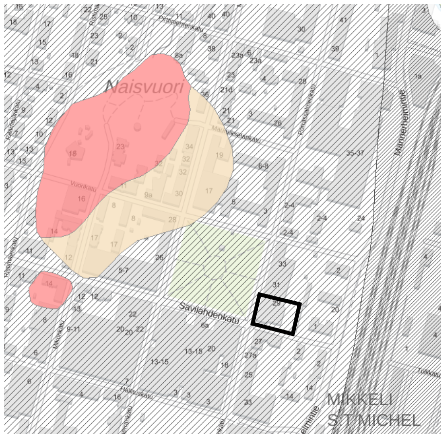
Kuva 4 Suunnittelualueen maaperä. Täytemaat on merkitty karttaan mustalla viivarasterilla, hiekka-moreeni beigellä väritäytöllä ja kallioma punaisella väritäytöllä. Suunnittelualueen sijainti on esitetty mustalla rajauksella. (Kartta: GTK:n Maankamara-palvelu)
