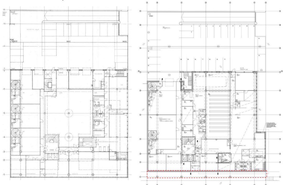
Kuva 11. (vas.) Yläkellarin pohjapiirustus, pääpiirustus, Arkkitetoimisto Eino Tuompo, Helsinki (1977 05 12). Kuva 12. (oik). Alakellarin nykytilanpohjapiirustus, Arkkitetoimisto Heikki Kirjalainen, 22.7.2009.
