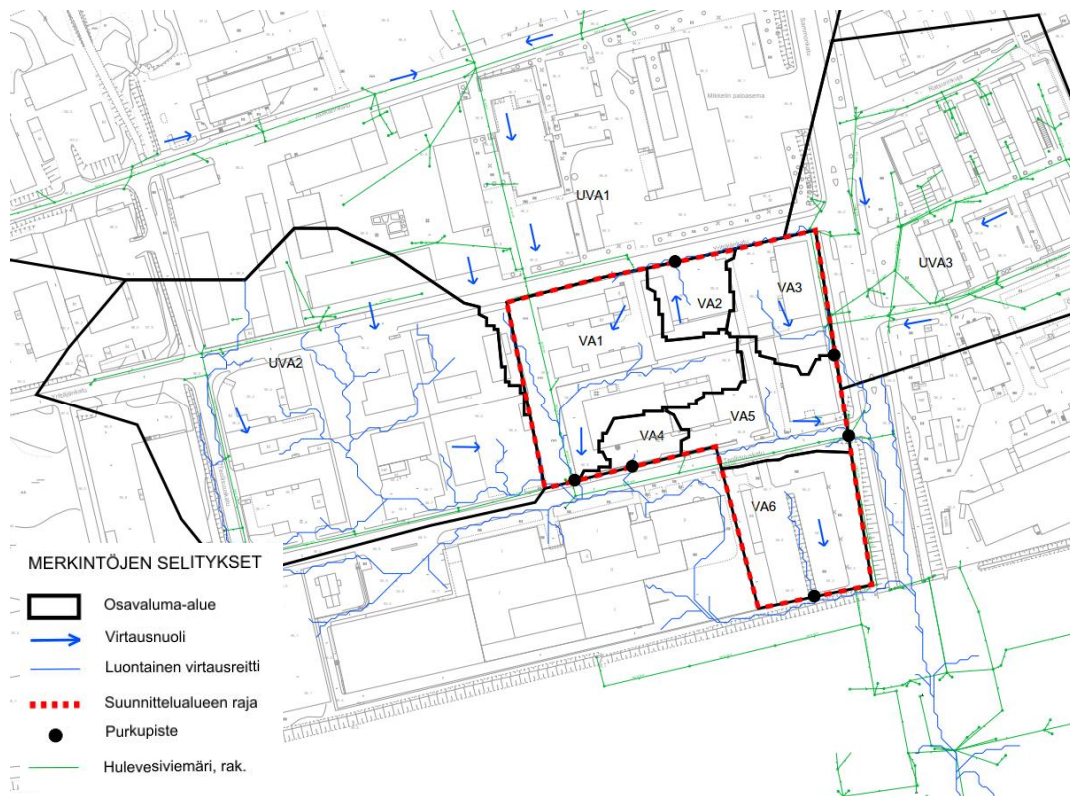
Kuva 6. Osavaluma-alueet VA1-VA6, ulkopuoliset osavaluma-alueet UVA1-UVA2 sekä hulevesien virtassuunnat niiden sisällä. suunnittelualueen rajaus on punaisella.
