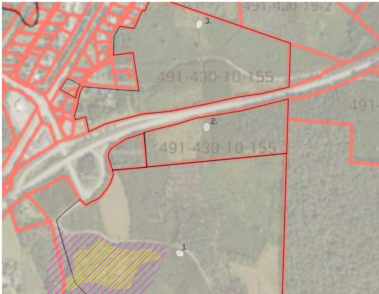
Kuva 9. Viivytyksaltaiden viitteelliset sijainnit merkattu valkoisella.
