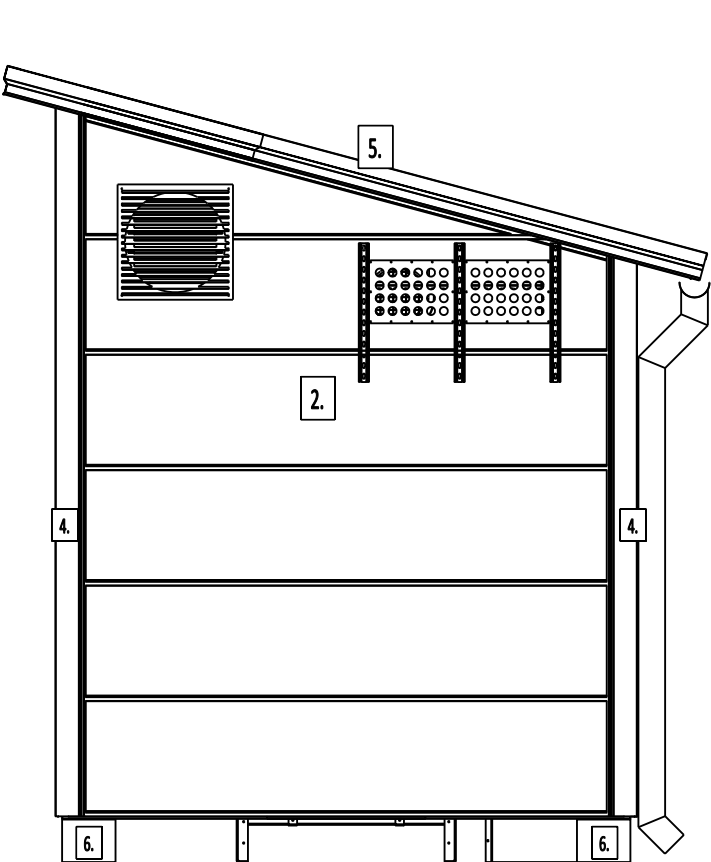
JULKISIVU C-D
