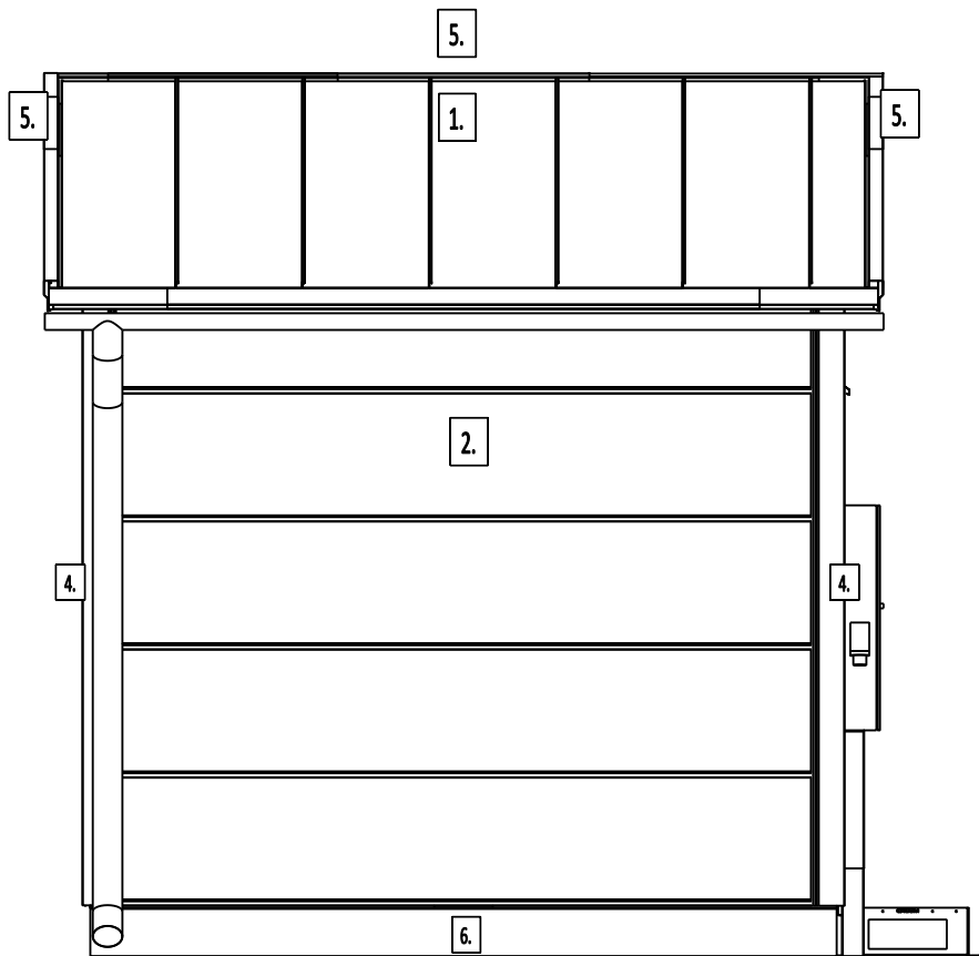
JULKISIVU B-C
