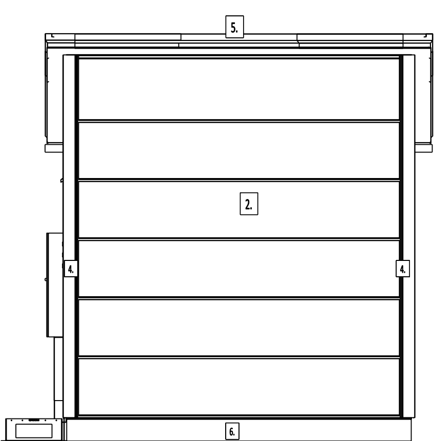
JULKISIVU A-D
