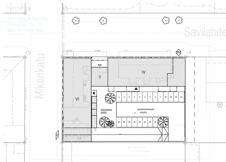
Kuva 14. Viitesuunnitelman asemapiirustus.
