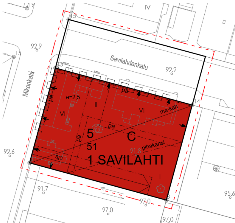
Kuva 11. Asemakaavaehdotuksen kaavakartta.
